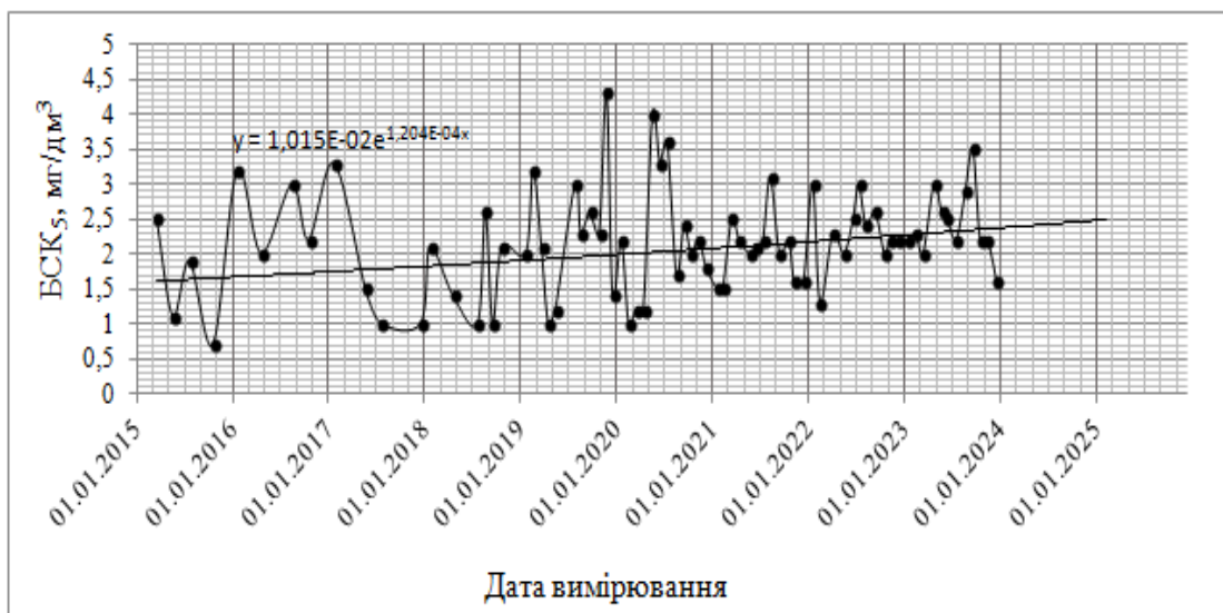
Рис. 1 - Часовий хід значень показника БСК 5 (р. Дунай, м. Кілія)
