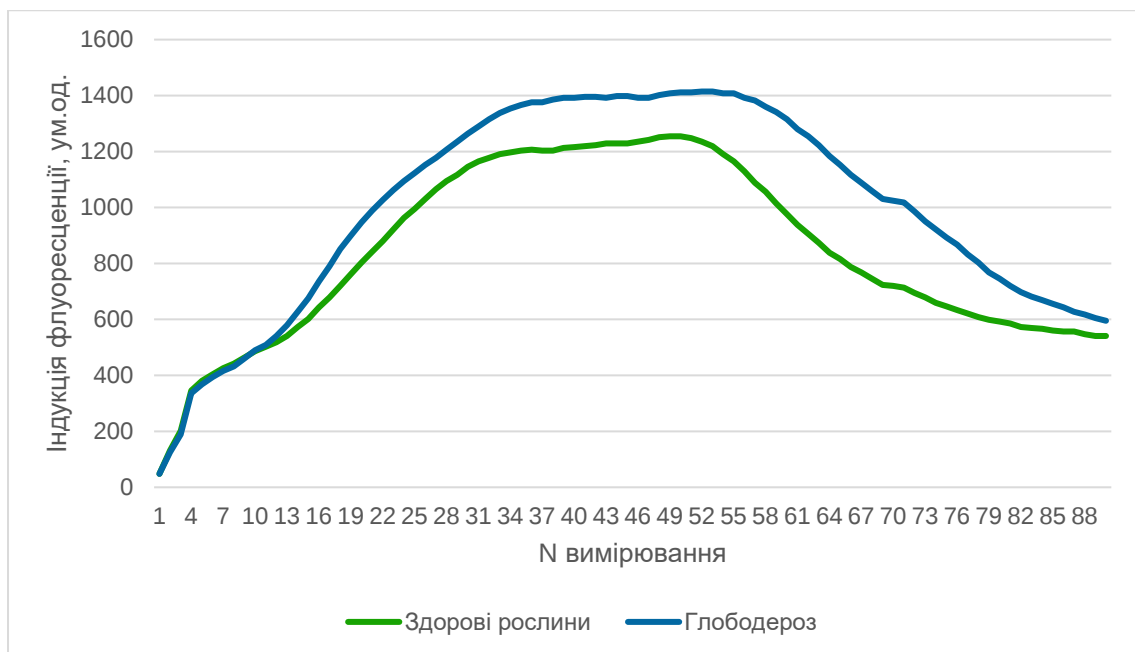
Рис. 1. Індукція флуоресценції хлорофілу в листках картоплі сорту Скрабниця за інвазії нематодами роду Globodera
