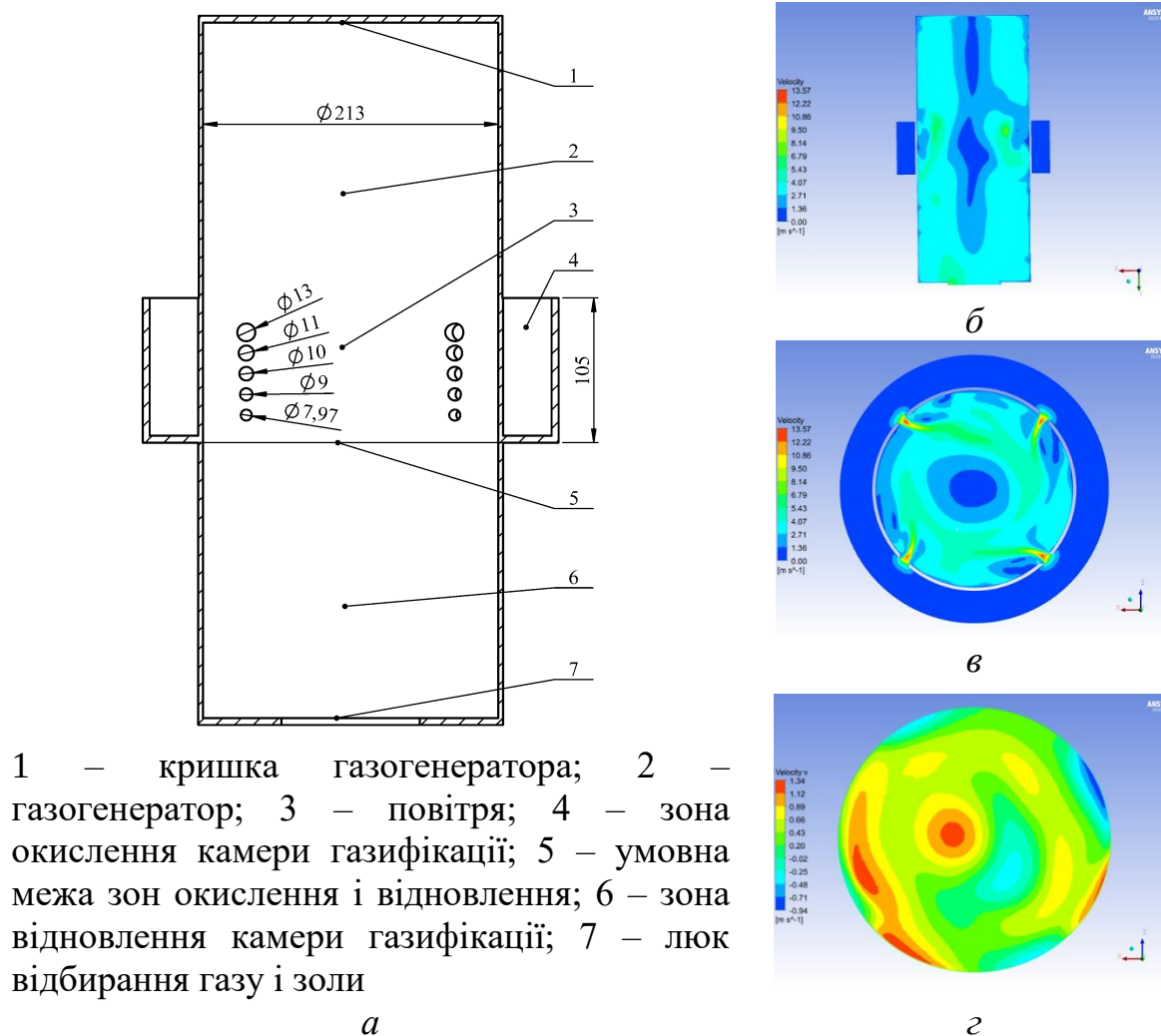
Рис. 2. Результати моделювання розподілу потоків повітря в газогенераторі, оснащеному газо-дутьтовим вузлом конструкції № 6: a – газогенератор; б – вертикальний переріз газогенератора; в – горизонтальний переріз, який проходить через центральний отвір зони окислення камери газифікації; г – переріз на вході в зону відновлення камери газифікації
