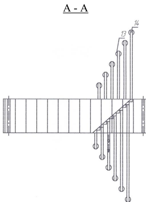
Рис. 2. Функціональна схема удосконаленої машини.
