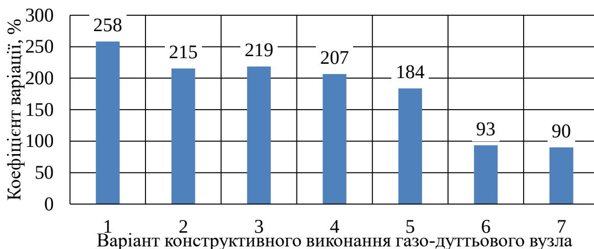
Рис. 1. Залежність коефіцієнту варіації від номеру конструктивного виконання газо-дутьового вузла газогенератора
