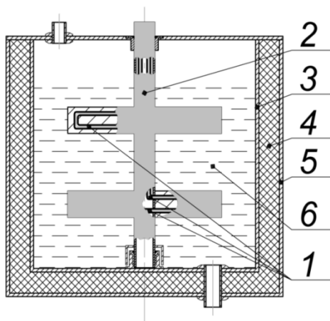
Рис. 1. Структурна схема електротепломеханічної системи для перемішування та підігріву субстрату у біогазовому реакторі [2]: 1 – електричний нагрівальний кабель; 2 – лопатева двоярусна мішалка з лопатями розміщеними під кутом; 3 – біогазовий реактор; 4 – утеплювальний матеріал; 5 – захисний металевий кожух; 6 – субстрат.
