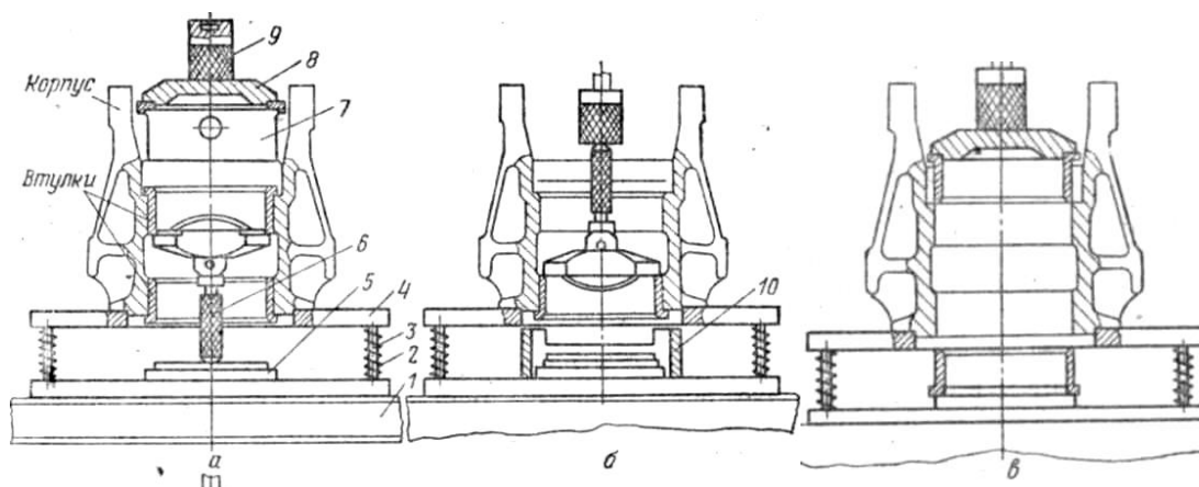
Рис. 1. Положення пристосування ОР-6305 при випресовуванні і запресовуванні втулок горизонтального шарніра: а – випресовування верхньої втулки; б – випресовування нижньої втулки; в – запресовування втулок: 1 – основа; 2 – пружина; 3 – штанга; 4 – плита; 5 – фіксатор; 6 – оправка; 7, 8 і 9 – наставки; 10 – підставка.
