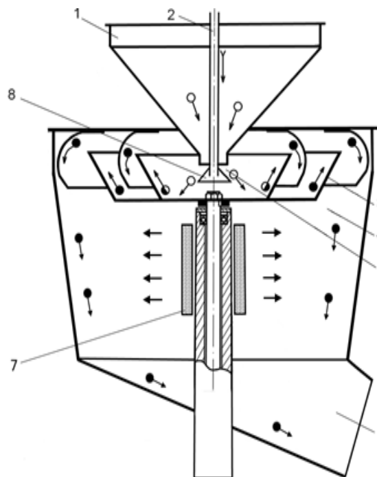
Рис. 1. Робочий процес модифікованого протруювача інерційно-фрикційного типу ПНУ-10: 1 – бункер; 2 – трубка подачі робочої рідини; 3 – чашоподібний змішувач; 4 – камера протруювання; 5 – дозатор насіння; 6 – вивантажувальна горловина; 7 – ультрафіолетовий електровипромінювач; 8 – конічний розподільник.
