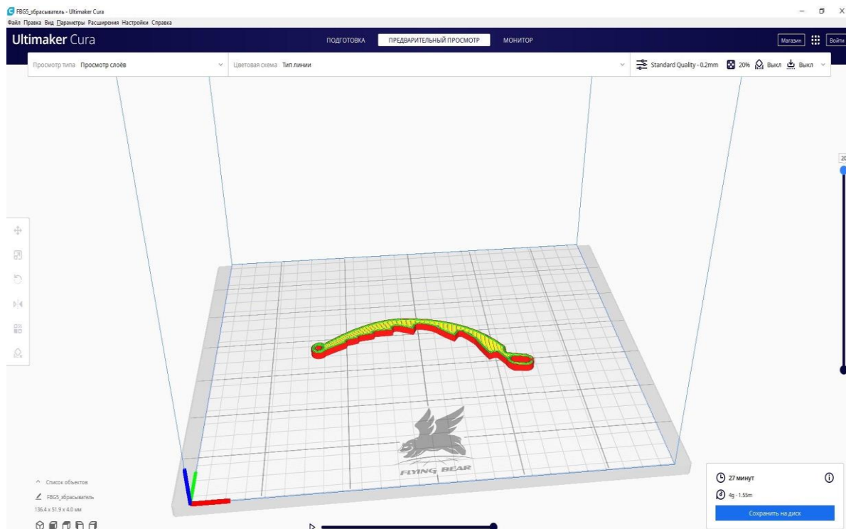
Рис. 2. 3D-модель гребінки-скидача висівального апарату у програмі “Cura”.
