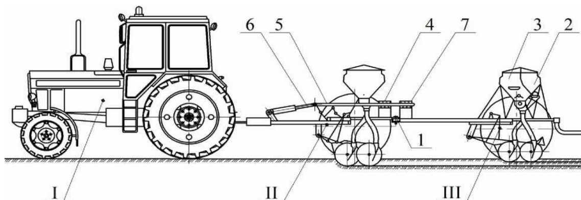
Рис. 1. Агрегат для внутрішньогрунтового мінерального удобрення та одночасної сівби зернових культур (вид збоку): I – трактор; II – машина для внесення основної дози мінеральних добрив; III – машина для сівби зернових та внесення стартової дози мінеральних добрив: 1 – шарнір; 2 – бункер для стартових добрив; 3 – бункер для насіння; 4 – направляючий елемент; 5 – блокуючий повзун; 6 – штанга; 7 – фіксуючий елемент.
