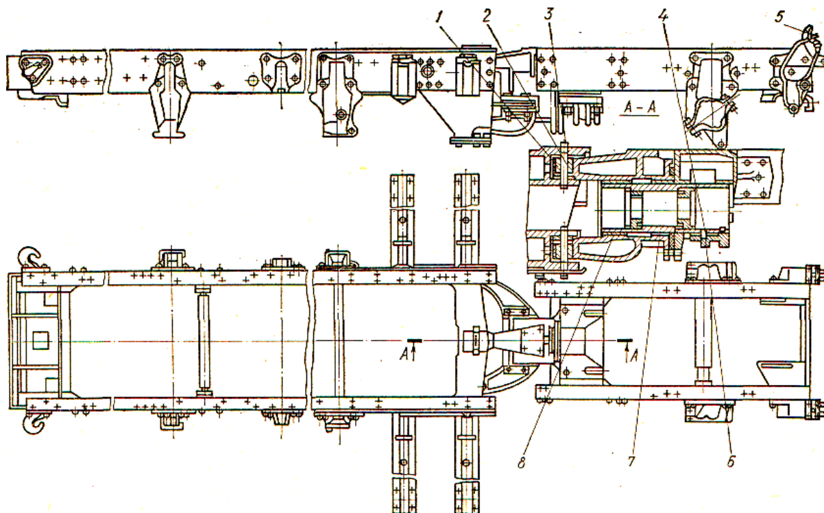
Рис. 2. Допустимі зазори (+) і натяги (—) в з'єднаннях під час ремонту рами трелювального трактора ЛТ-171(мм): 1 – корпус-втулка -0,02; 2 – втулка-вісь +1,30; 3 – опора-вісь +0,40; 4 – труба-штифт +0,50; 5 – кронштейн-штифт -0,01; 6 – бугель-штифт +0,01; 7 – втулка-труба +2,5; 8 – корпус-втулка -0,02.
