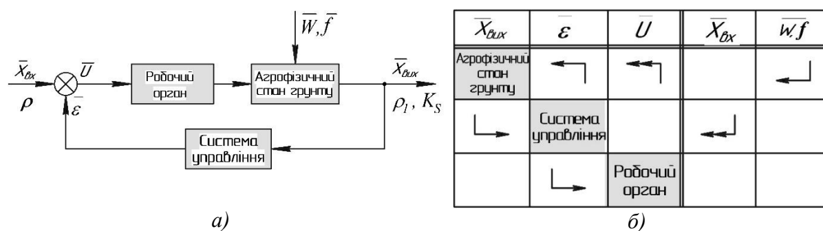
Рис. 1. Модель потокової системи управління обробітком ґрунту.
