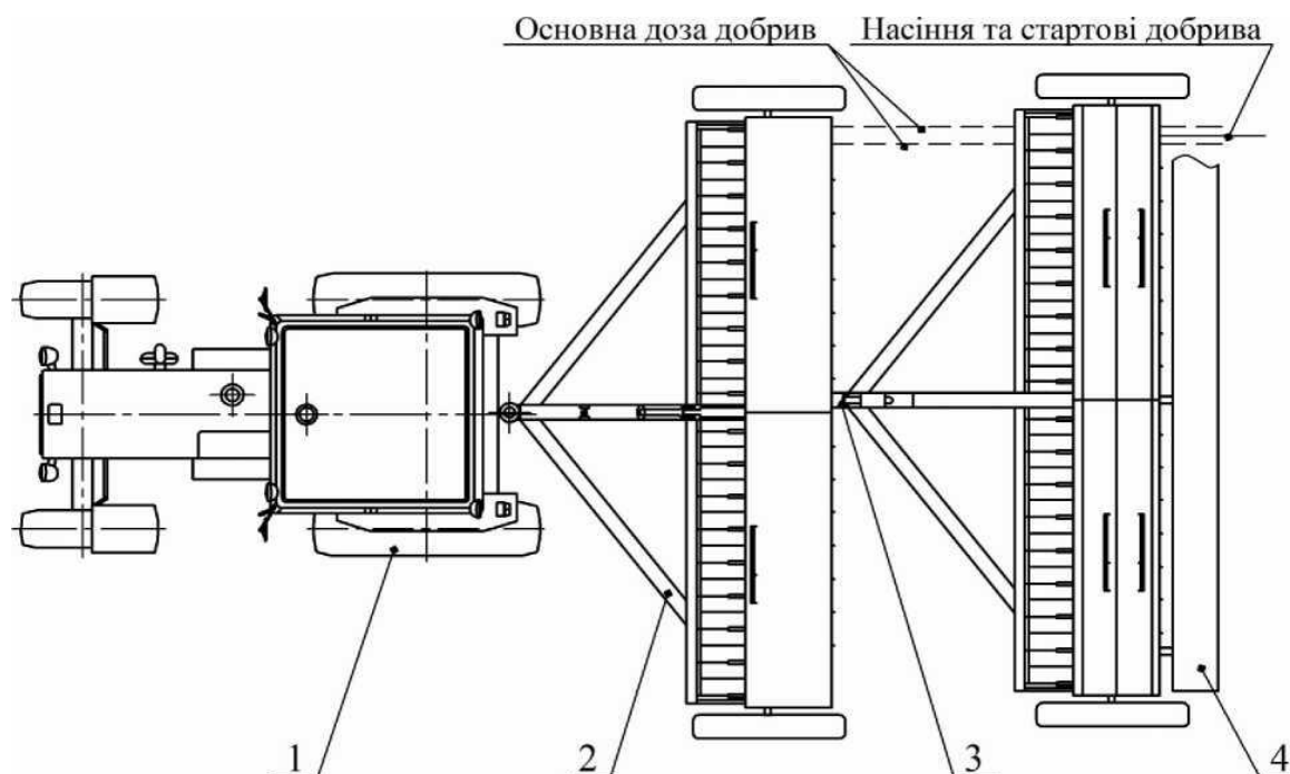
Рис. 2. Комбінований удобрювально-посівний машинно-тракторний агрегат (вид зверху): 1 – колісний агрегатуєчий трактор; 2 – сівалки для внесення у ґрунт основної дози мінеральних добрив стрічковим способом; 3 – начіпний пристрій; 4 – сівалка зернових культур з пристроєм для одночасного внесення у ґрунт стартової дози мінеральних добрив.
