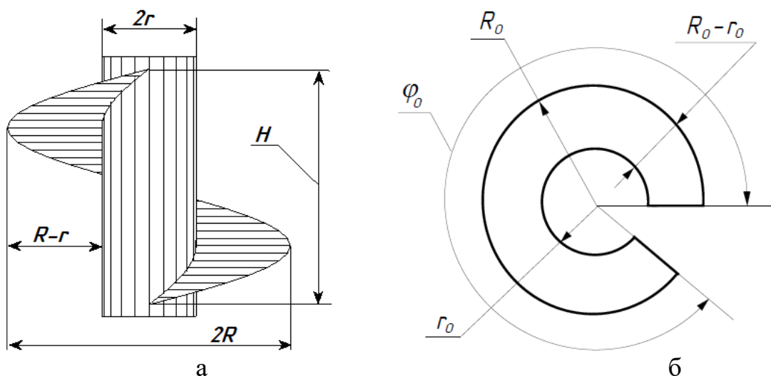
Рис. 1. Графічні ілюстрації до побудови умовної розгортки витка шнека: а) фронтальна проекція витка із зазначеними розмірами; б) умовна розгортка витка.
