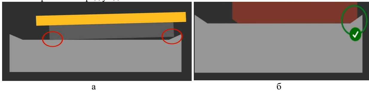
Рис. 3. Контакт нової удосконаленої колодки та зношеного диска: а) контакт традиційної колодки та зношеного диска б) контакт удосконаленої колодки та зношеного диска
