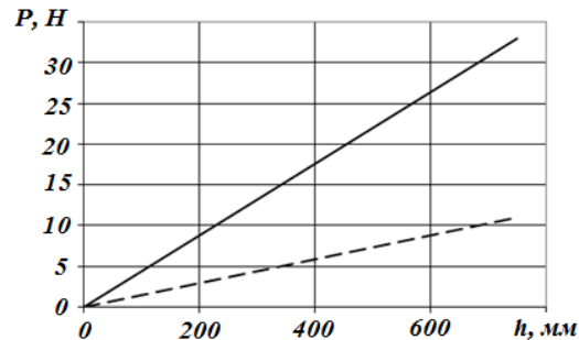
Рис. 2. Залежність сили P , що діє на плоди, від висоти шару плодів h : ____ - статична сила; _____ - сума статичних і динамічних сил.
