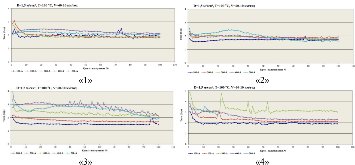
Рис. 5. Результати зносних гальмувань на швидкості 10-60 км/год Джерело: складено автором на основі протоколів випробувань
