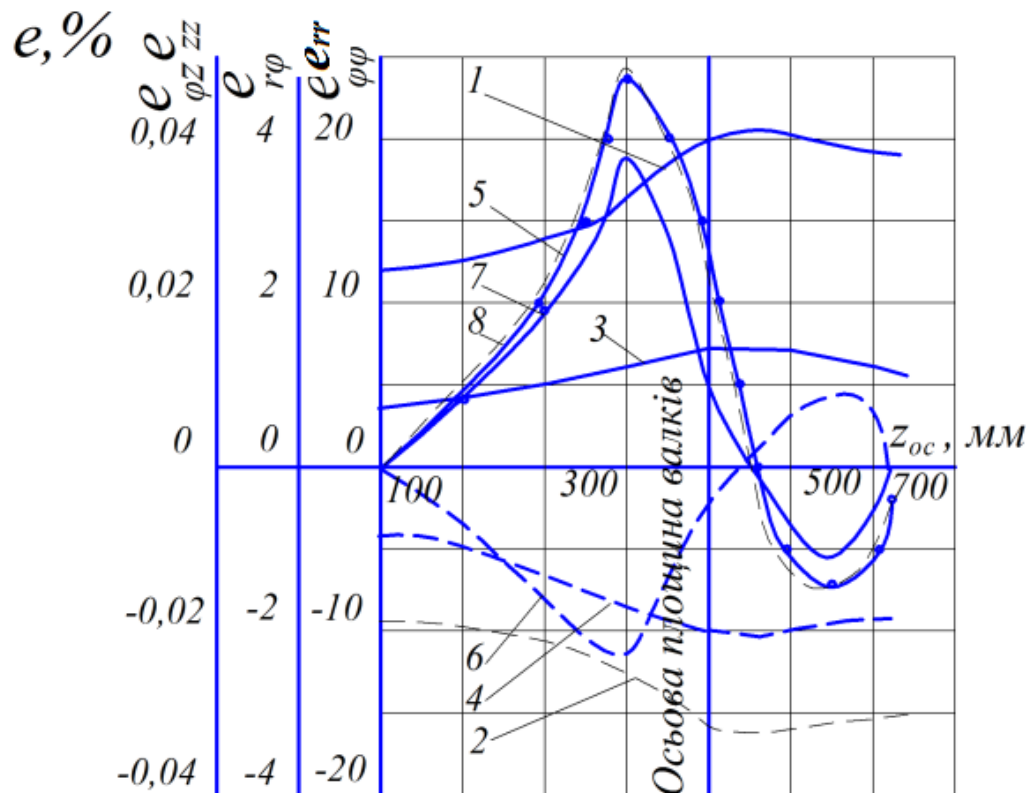
Рис. 2. Графіки зміни компонентів тензора деформацій e_{\phi\phi} (1, 2), e_{\phi r} (3, 4), e_{\phi z} (5, 6) і e_{zr} (7, 8) металу місця вигину швелера 150 \times 100 \times 2 мм уздовж ділянки плавного переходу в третій формувальній клітці ( 30 - 50^\circ ) на зовнішній (1, 2, 5, 7) і внутрішній (2, 4, 6, 8) поверхнях
