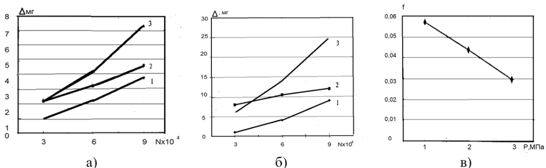
Рис. 5. Залежність зносу ролика (а) та вкладиша (б) від числа циклів та питомого тиску: 1- P=1,34 МПа; 2- P=1,98 МПа; 3- P=2,94 МПа; в - залежність коефіцієнта тертя наплавленої алюмінієвої бронзи Бр Амц 9-2 від питомого тиску.
