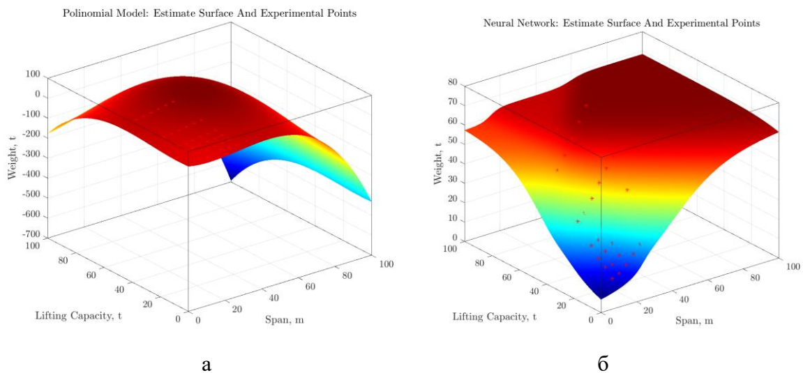
Рис. 8. Порівняння результатів розрахунку маси крану групи режимів роботи А6-А8 в залежності від прольоту і вантажопідйомності на основі функціональної залежності і за допомогою нейромережі: а – розрахунок на основі функціональної залежності; б – розрахунок за допомогою нейромережі
