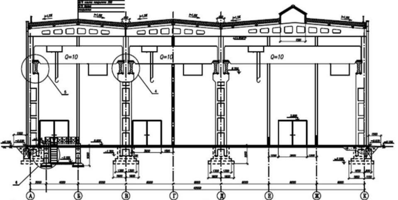
Высот 5 1:20
