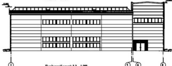
Поперечный разрез 2-2 1:200
