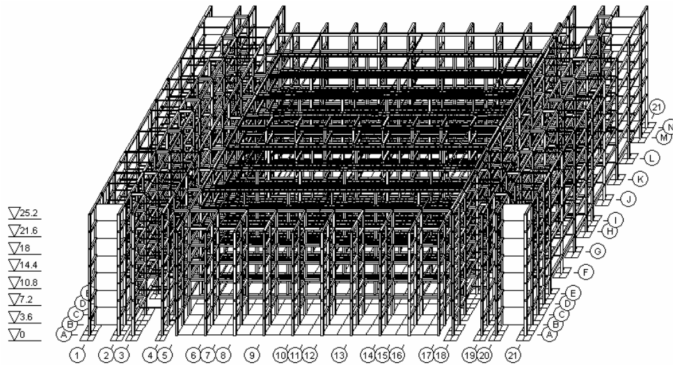
Тектонічне формоутворення об'ємно-планувальної структури зв'язкової конструктивної схеми типової серії 1-020-1/83 із уніфікованих конструктивних елементів
