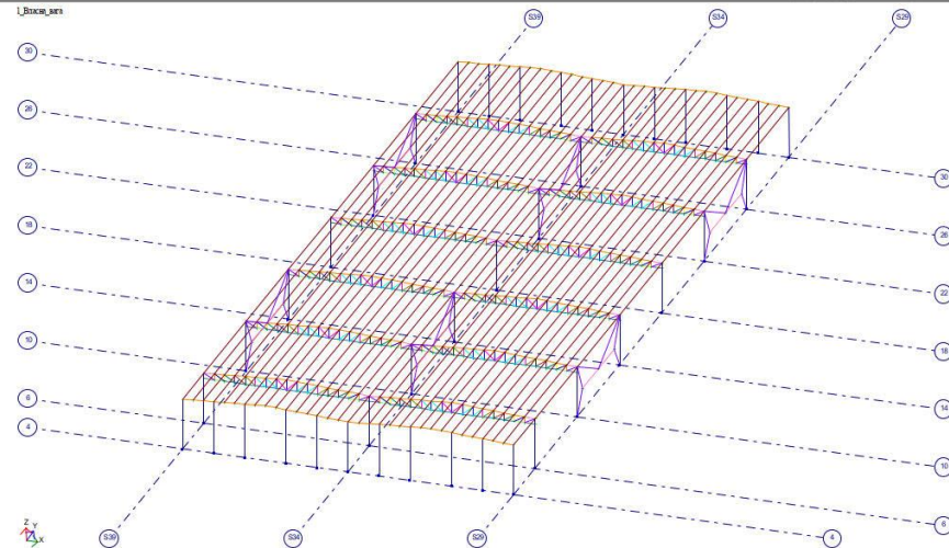
Колірне відображення конструктивних елементів
