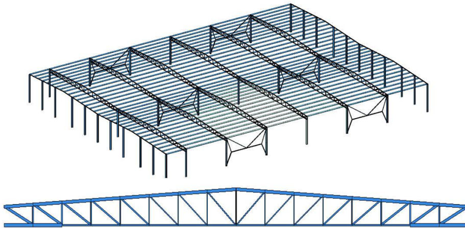
3D модель. Рамно-зв'язкова конструктивна схема будівлі виробничого призначення
