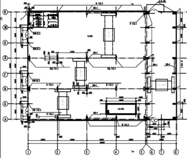
План производственного здания 1:200
