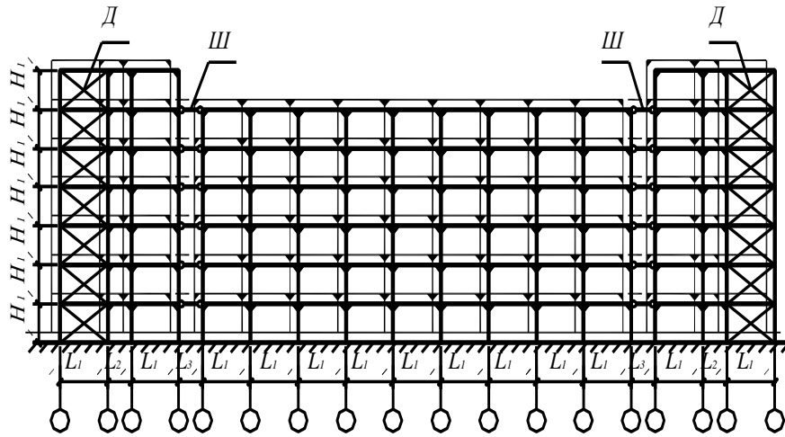
Типова зв'язкова конструктивна схема багатоповерхової будівлі виробничого призначення
