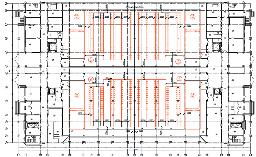
Планувальне рішення будівлі виробничого призначення
