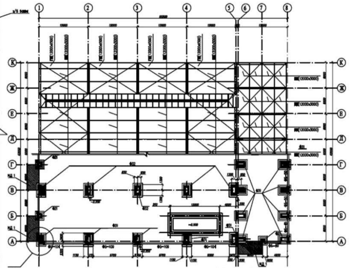
План фундамента и перегородки 1:200
