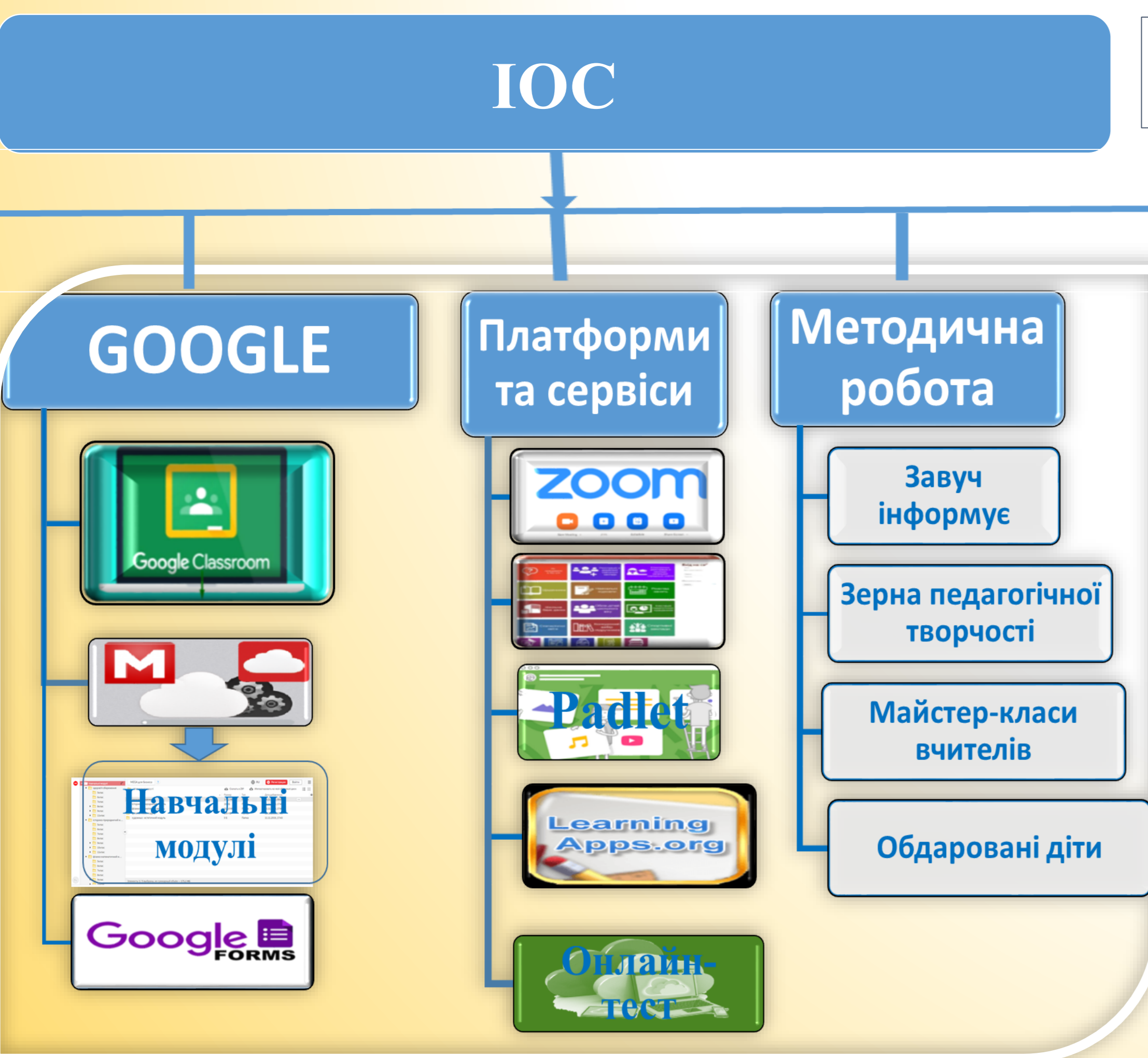
Рис.3 Структура ІОС
