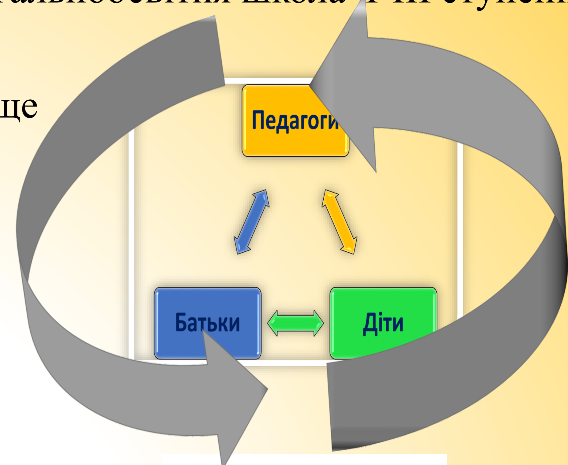
Рис.1 Модель ІОС
