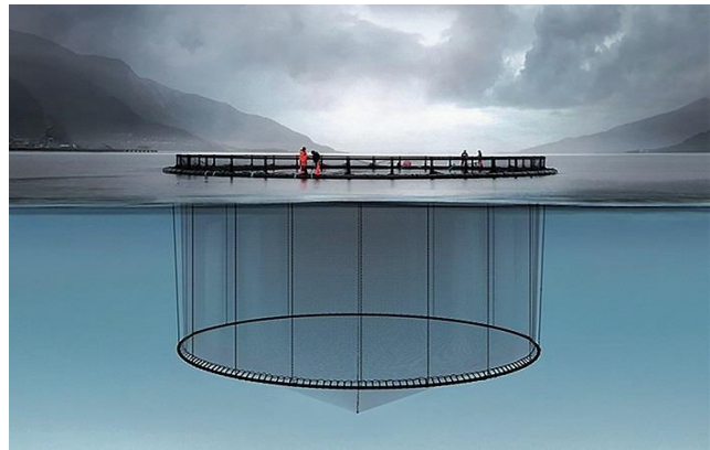
Рис. 5. Круглі морські пластикові садки
