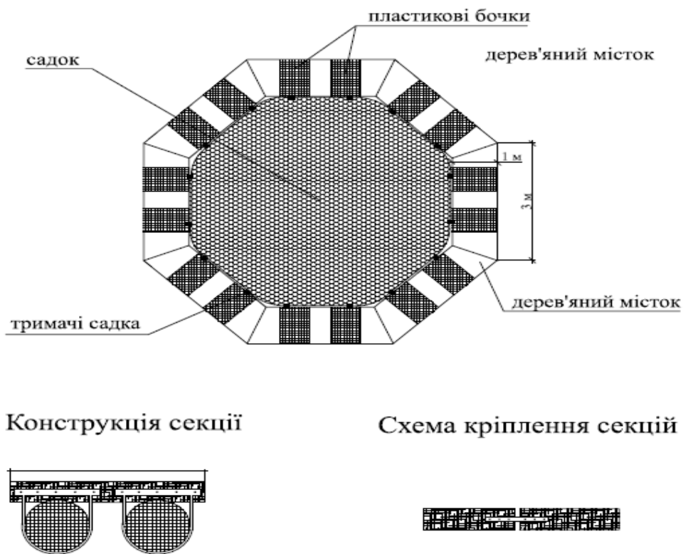
Рис. 2. Будова восьмигранного садка
