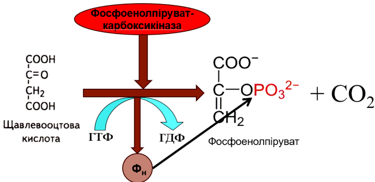
Рис. 2.39. Декарбоксілювання та фосфорилування оксалоацетату до фосфоенолпірувату
