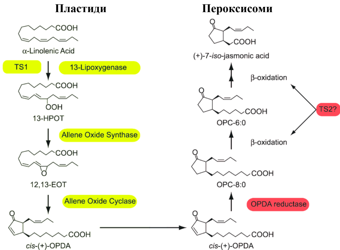
Рис. 3.14. Біосинтез жасмонової кислоти
