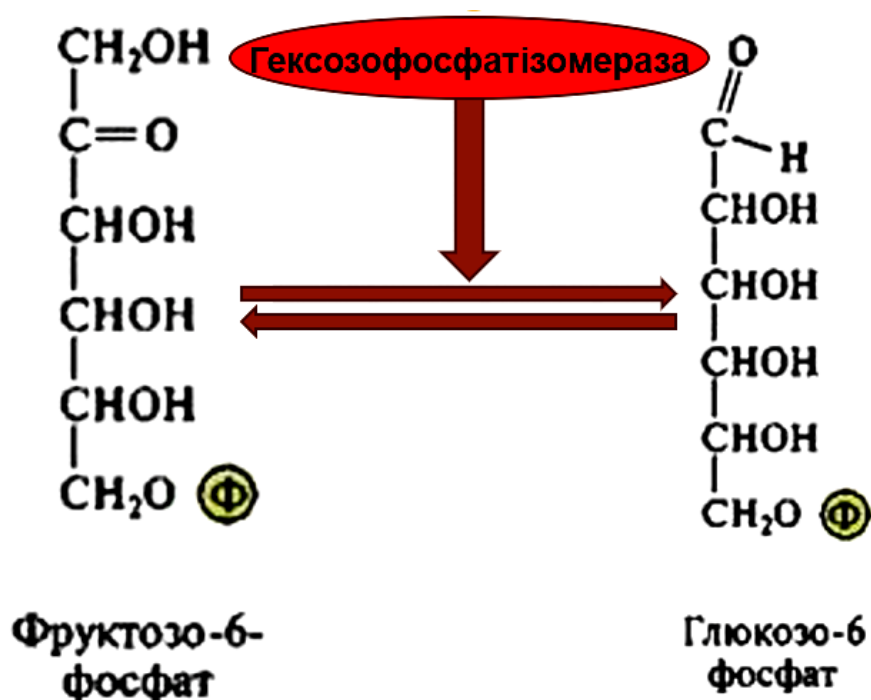
Рис. 2.47. Ізомеризація фруктозо-6-фосфату
