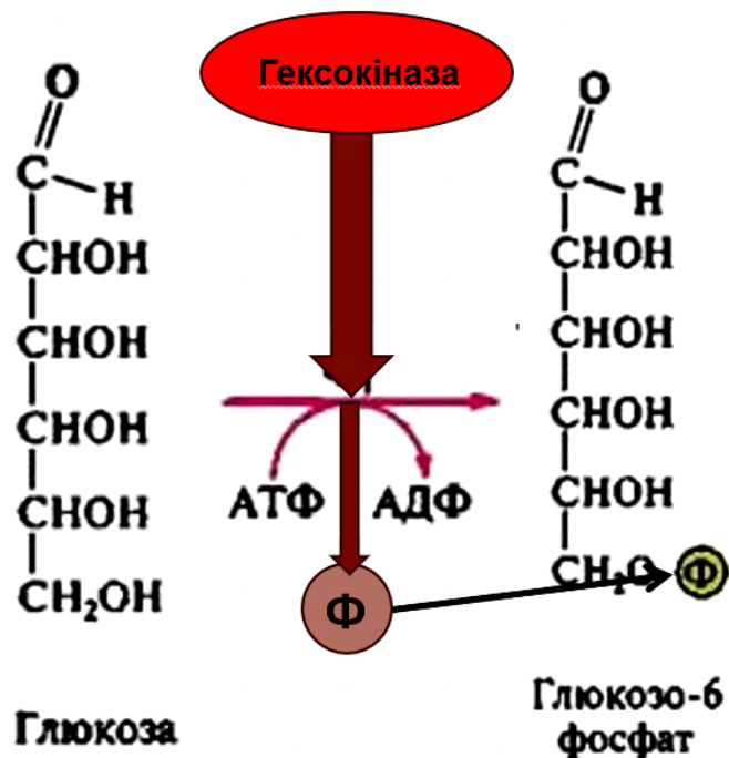
Рис. 2.1. Фосфорилювання глюкози до глюкозо-6-фосфату
