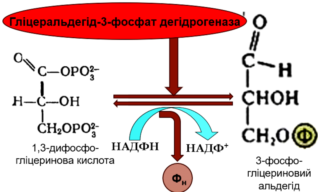
Рис. 2.43. Утворення 3-фосфогліцеринового альдегіду
