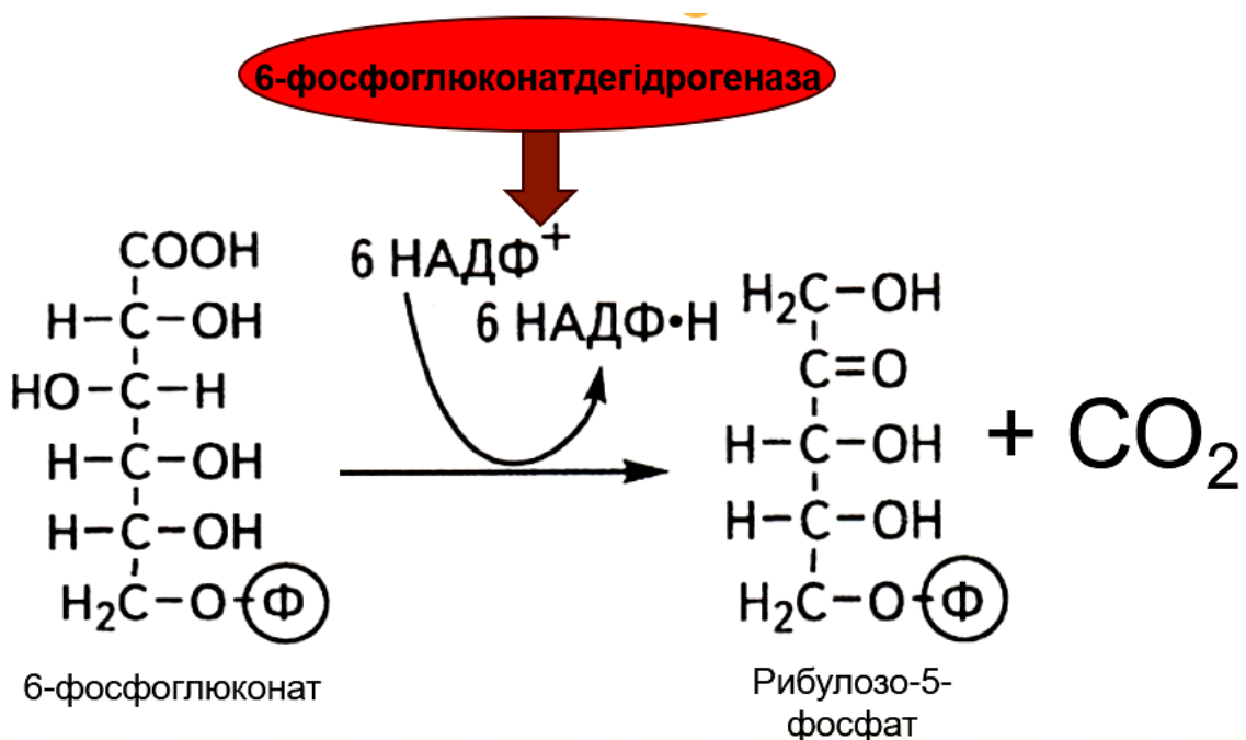
Рис. 2.24. Реакція окисного декарбоксилування 6-фосфоглюконату з утворенням неорганічного CO 2 і пентози
