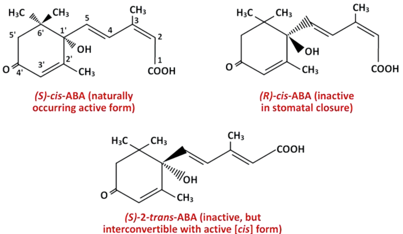
Рис. 3.10. Будова абсцизової кислоти
