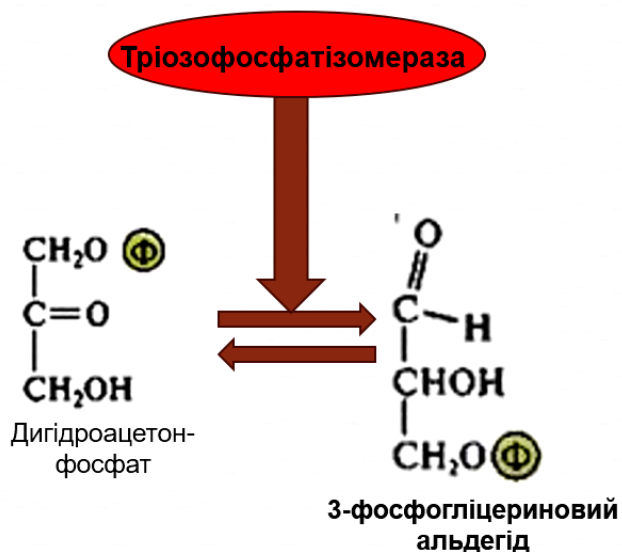
Рис. 2.5. Взаємоперетворення фосфотріоз (фосфодиоксиацетону і 3-фосфогліцеринового альдегіду)
