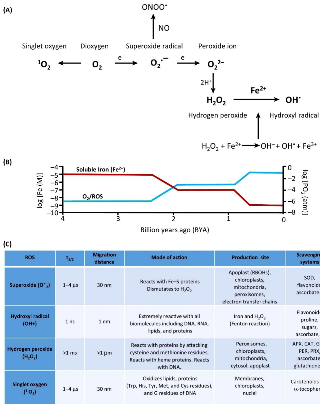
Рис. 6.9. Схема утворення різних форм вільних радикалів
