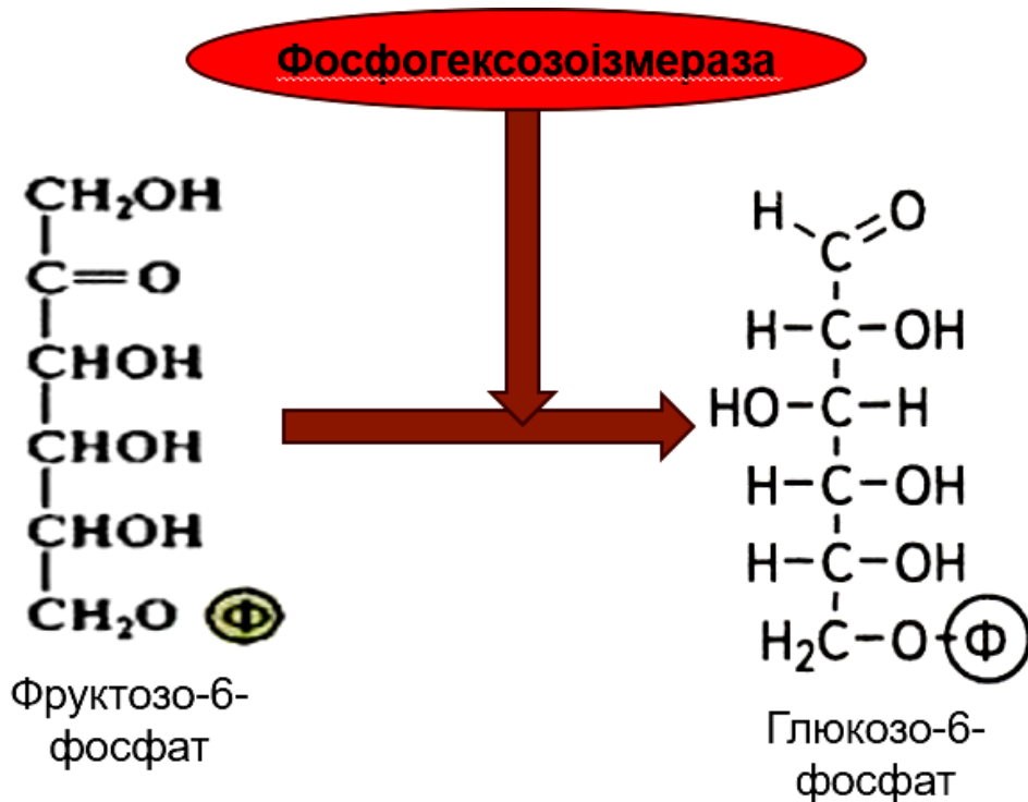
Рис. 2.30. Ізомеризація фосфогексоз
