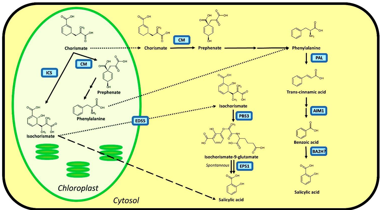
Рис. 3.15. Можливі шляхи біосинтезу СА в рослинах
