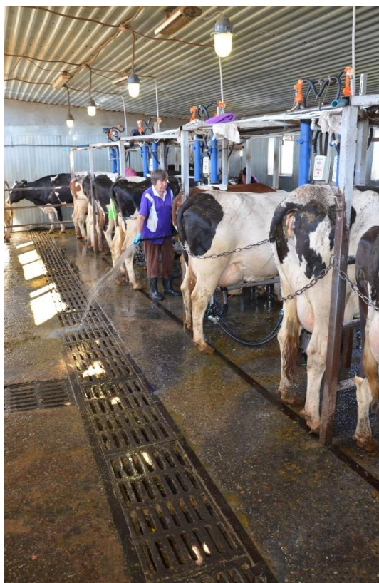
Рис. 1.3.10. Каналізаційний жолоб установки прохідного типу на 12 місць (АФ „Піщанська” Харківської області).
