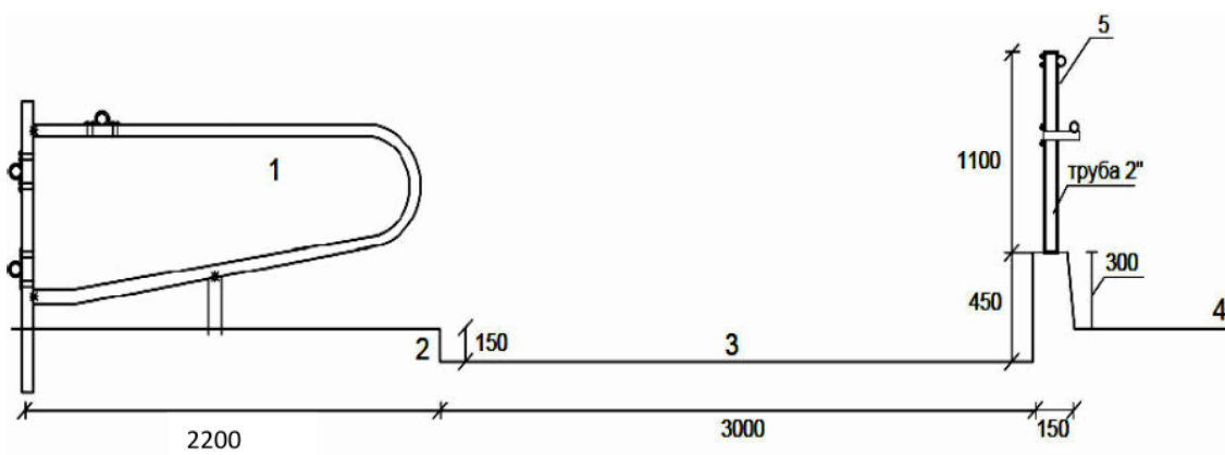
Рис. 1.1.6. Конструктивне рішення боксу, прогулянкової алеї та обмежувального бордюру (від франц. Bordure – край, борт) кормового столу.
