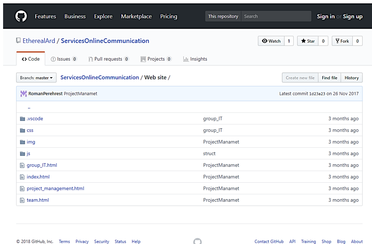
Рис. 3 – Фрагмент репозитарію
