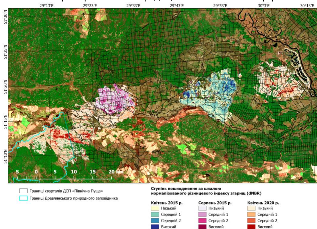
Рис. 3. Пожежі у зоні відчуження у 2015 р. (квітень – відтінки синього, серпень - відтінки фіолетового) та у 2020 р. (відтінки червоного).
