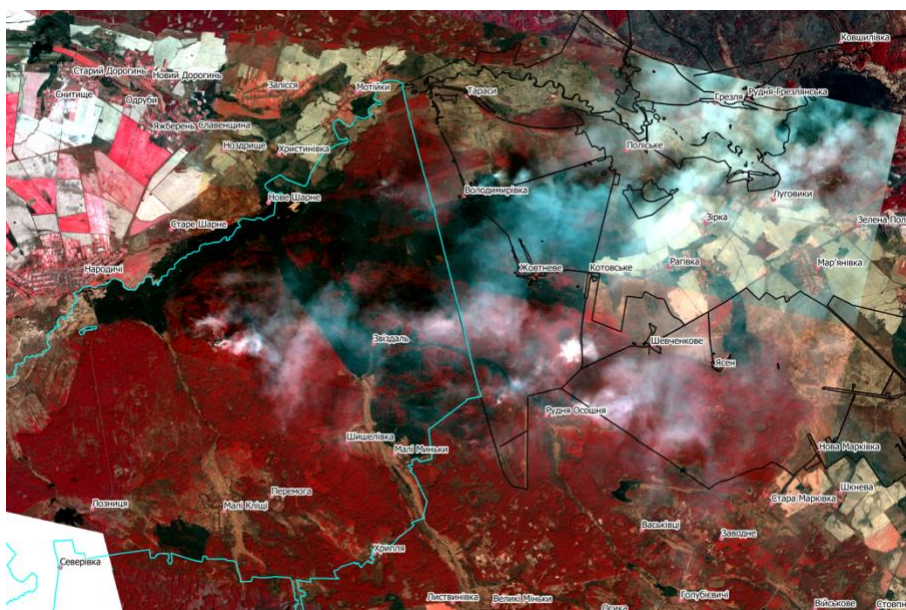
Рис. 3. Композитний знімок PlanetScope території розвитку пожежі 3-7 квітня 2020 р у західній частині зони відчуження.
