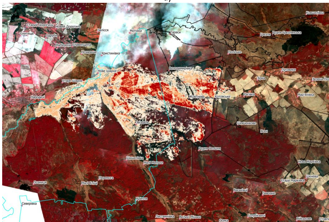
Рис. 4. Інтенсивність вигорання території за показником dNBR станом на (знімок PlanetScope): а) 5 квітня 2020 р. (червоне – зони інтенсивного горіння - лісові пожежі)
