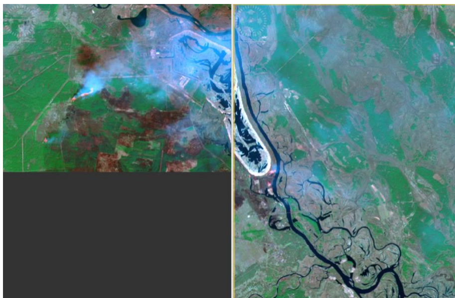
Рис. 6 Розвиток пожежі у 10-км зоні зони відчуження станом на 12 квітня.
