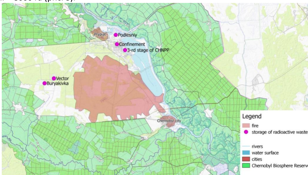
Рис. 2. Контури пожежі у 10-км зоні зони відчуження (рожевий) протягом 8-12 квітня 2020 р. Темно зелений колір - Чорнобильський радіаційно-екологічний біосферний заповідник.
