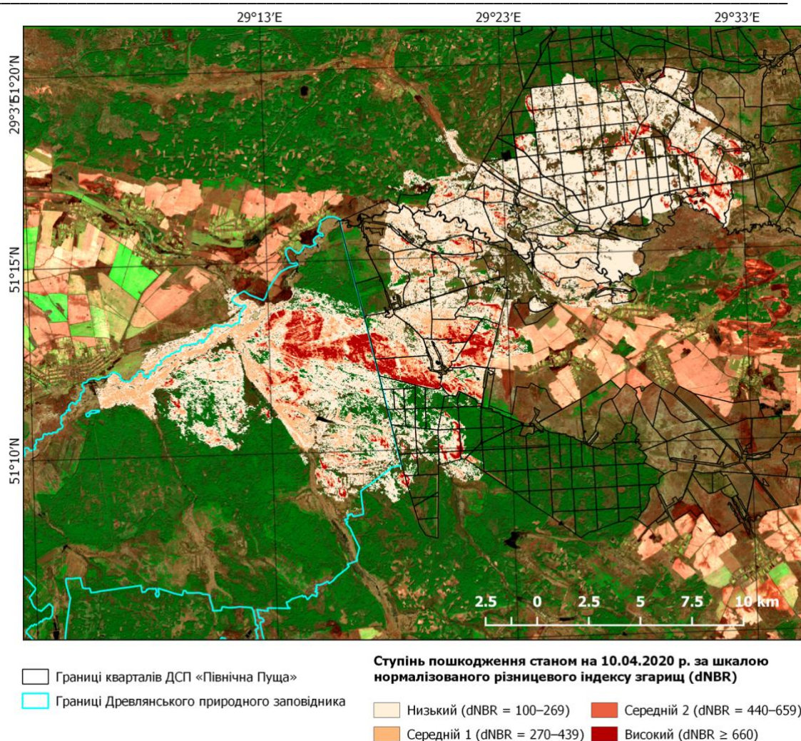
Рис. 2. Природна пожежа 3-10 квітня 2020 р. у районі населених пунктів Народичі-Поліське, якою пройдено територію Древланського природного заповідника та зони відчуження. Загальна площа пожежі 3-10 квітня – 19200 га, в тому числі - Древланський природний заповідник – 6000 га, зона відчуження -11500.
