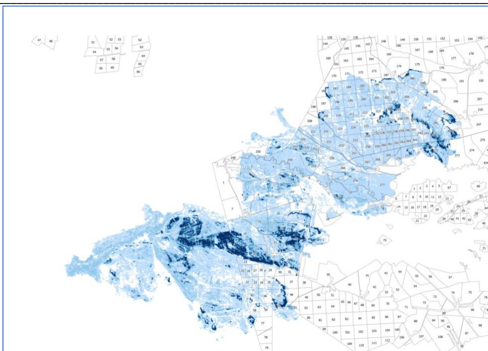
Рис. 3. Розвиток пожежі 5-10 квітня 2020 р. та її інтенсивність на території Котовського та Денисовецького лісництв ДСП «Північна Пуша»
