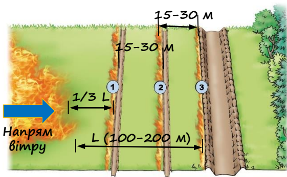
Рис.7. Ступінчастий відпал
