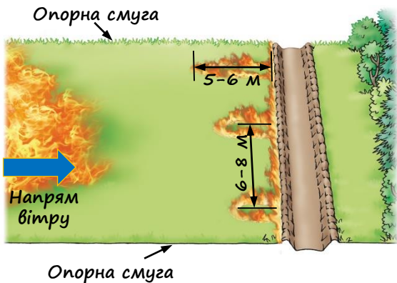
Рис.8. Відпал способом гребінки
