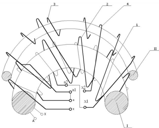
Рис. 1. Конструктивне виконання зварювального трансформатора.
