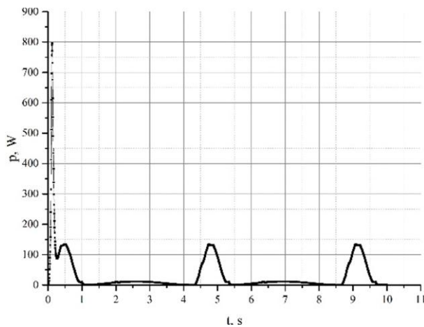
Рис. 2. Миттєва потужність теплових втрат.
