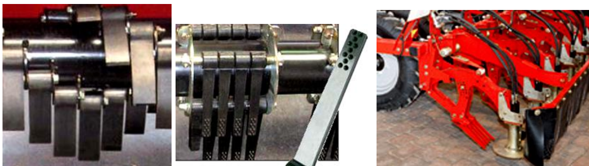
Рис. 1. Робочі органи гичковідокремлювальної машини VM 330: а – роторний гичкоріз, б – поліуретанові бичі на валах, що зустрічно обертаються, в – копірний дообрізкач активного типу.
