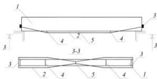
Рис. 5. Влаштування шпренгельних затяжок:
