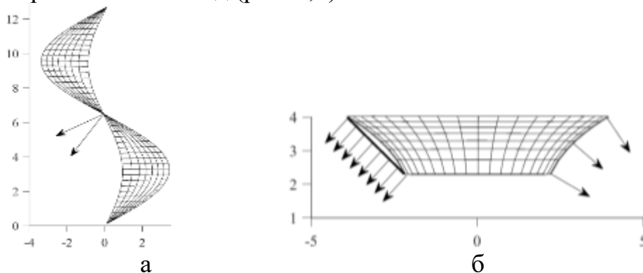
Рис. 1. Зображення витка гвинтового коноїда:
