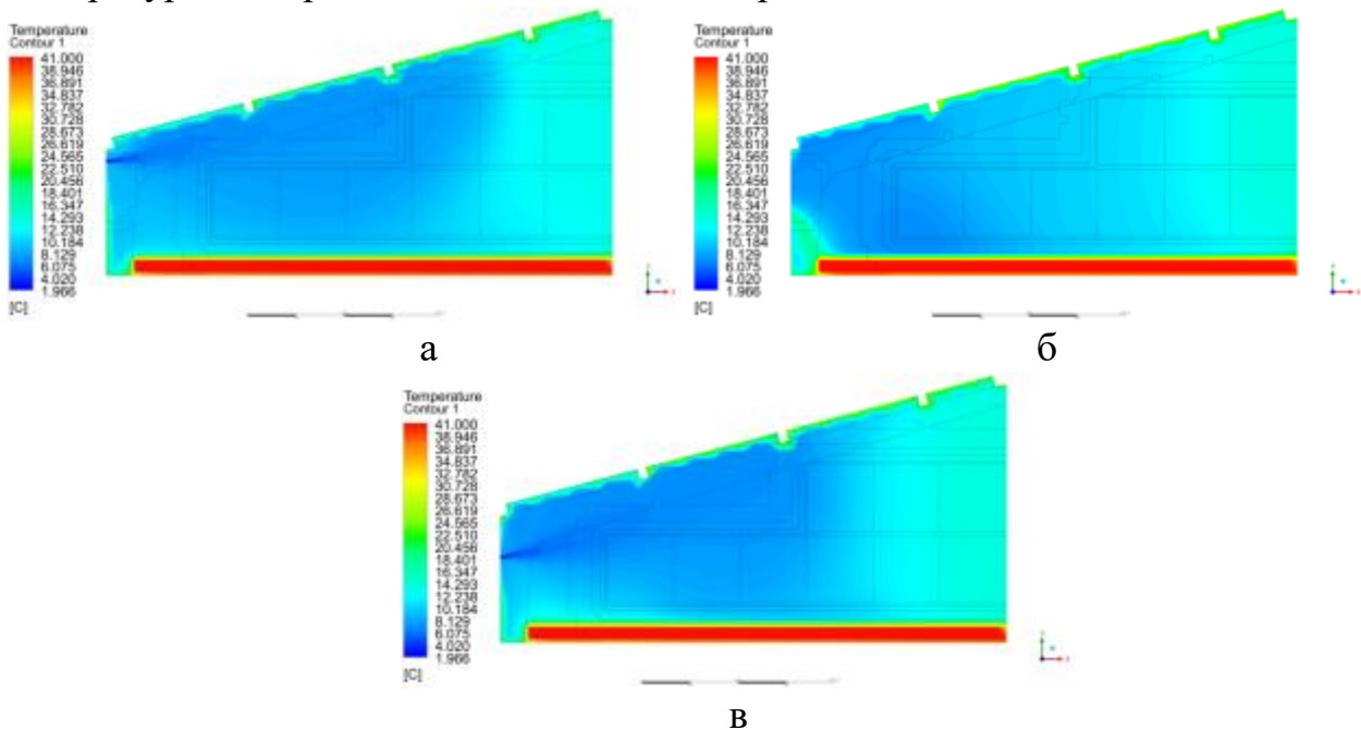
Рис. 1 – Поле температур ( ^{\circ}\text{C} ) в приміщенні пташника на відстані від передньої торцевої стінки на: а – 16,23 м.; б – 50,78 м.; в – 85,25 м.
