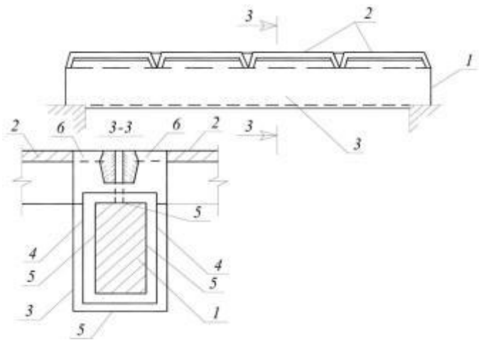
Рис. 4. Влаштування залізобетонної обойми:
