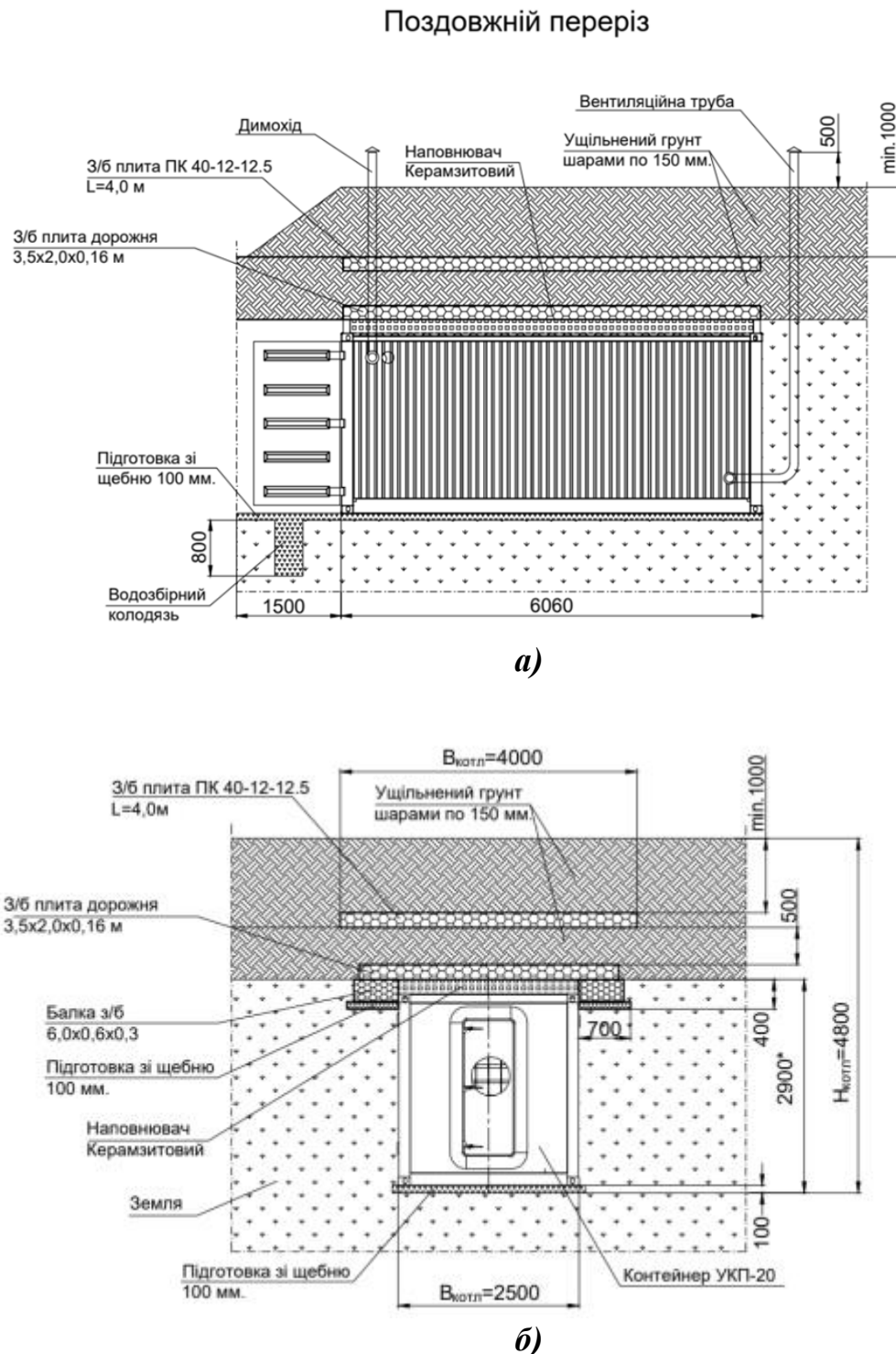
Рис. 1. Схема захисної споруди у складі: каркасний модульний будинок із захисним багатошаровим покриттям; а – поздовжній переріз; б – поперечний переріз
