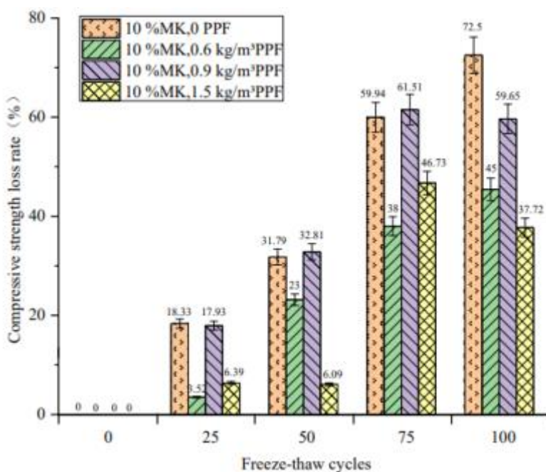
Рис. 1. Зв'язок між циклами заморозування–відтавання та швидкістю втрати міцності на стиск під час багатосолевого впливу та циклів заморозування–відтавання для PPF [3]
