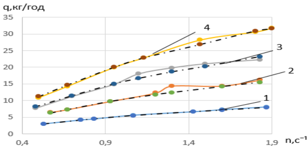
Рисунок 4 - Вплив частоти обертання ( n ) на продуктивність дозатора: (1, 2, 3, 4 – відповідно 2, 4, 6, 8 отворів;)
