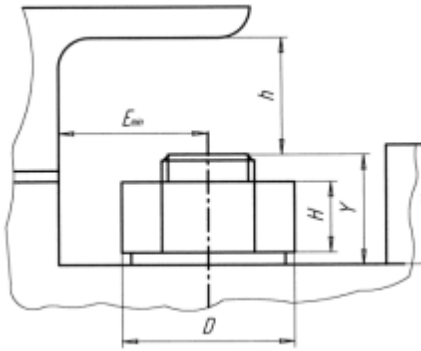
Рисунок 2 – Схема для вибору головок і кільцевих ключів на вузла для визначення параметрів підставі доступності
