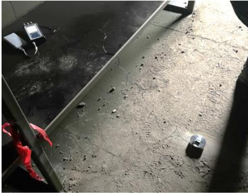
Рис. 2. Розташування трьохкомпонентного датчика вібрації
