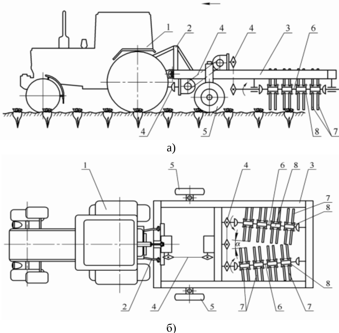
Рис. 1. Конструктивно-технологічна схема двохвального очисника головок коренеплідних культур від залишків гички на корені:
