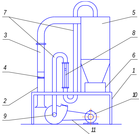
Рис. 1. Принципова схема та загальний вигляд парусного класифікатора.
