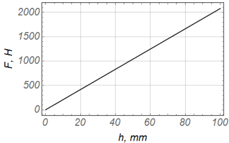
Рис. 1. Залежність зміни зусилля пружини від переміщення
