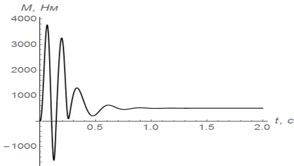
Рис.1. Графік зміни моменту в пружному елементі, що з'єднує привод з робочим органом конвеєра
