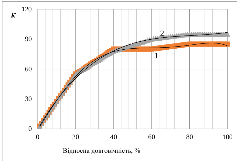
Рис. 2. Кінетичні характеристики накопичення втомного пошкодження зразків Ст 20 (1 – графік розраховано за експериментальними даними; 2 – апроксимація степеневою функцією)
