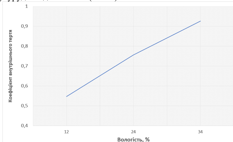
Рис. 1. Коефіцієнт внутрішнього тертя кукурудзи в залежності від вологості
