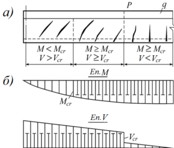
Рис. 1. До класифікації тріщин: a – граничні умови виникнення тріщин; б – епюри зусиль; M і V – максимальні значення згинального моменту і поперечної сили на ділянці, що розглядається [1]
