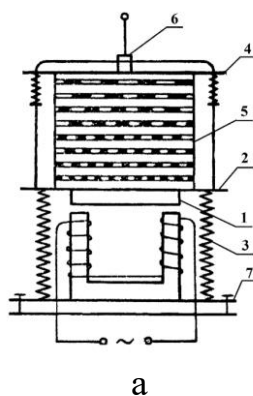
Рис. 2. Вібраційно-решітний класифікатор РКФ-1: а – функціональна схема; б – набір решіт.
