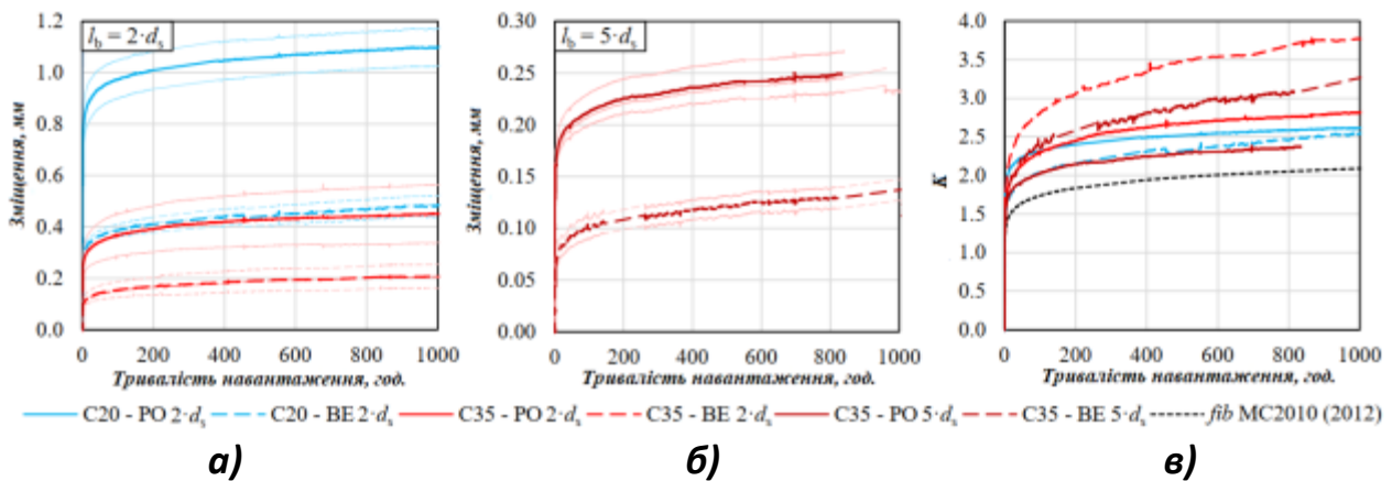
Рис. 3. Збільшення проковзування арматури при дії довготривалого навантаження для різних випробувань та класів бетону (РО – висмикування, БЕ - балочне) [5]:
