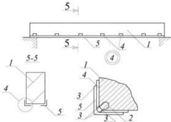
Рис. 3. Влаштування металевих кутиків:
