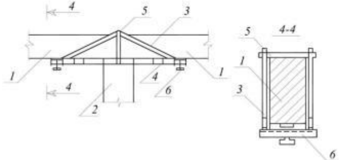
Рис. 6. Підведення кронштейнів, які розвантажують конструкцію:
