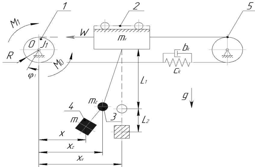
Рис. 1. Розрахункова динамічна модель системи «візок-вантаж»
