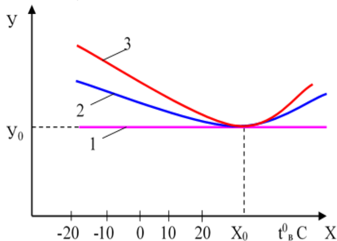
Рис. 3 – Графік інтенсивності зношування агрегатів автотранспорту залежно від температури навколишнього середовища, X = t_s
