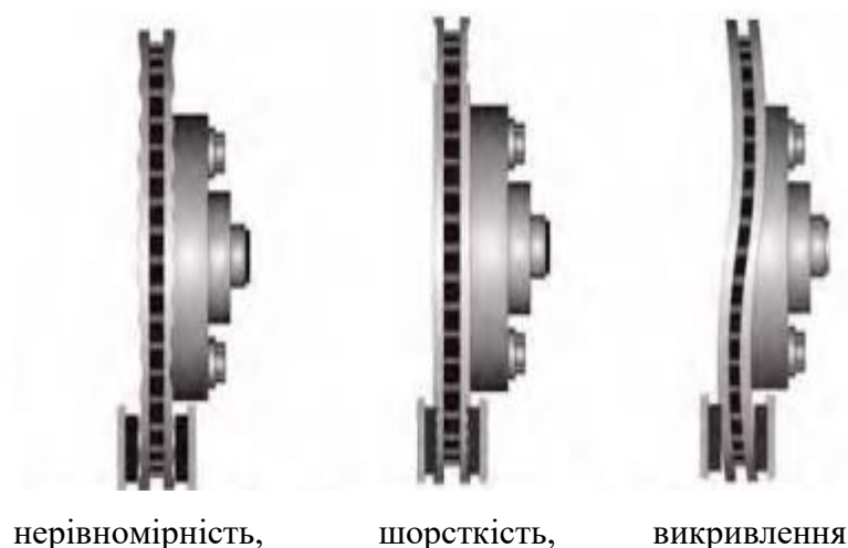
Рис. 1 – Основні дефекти дисків
