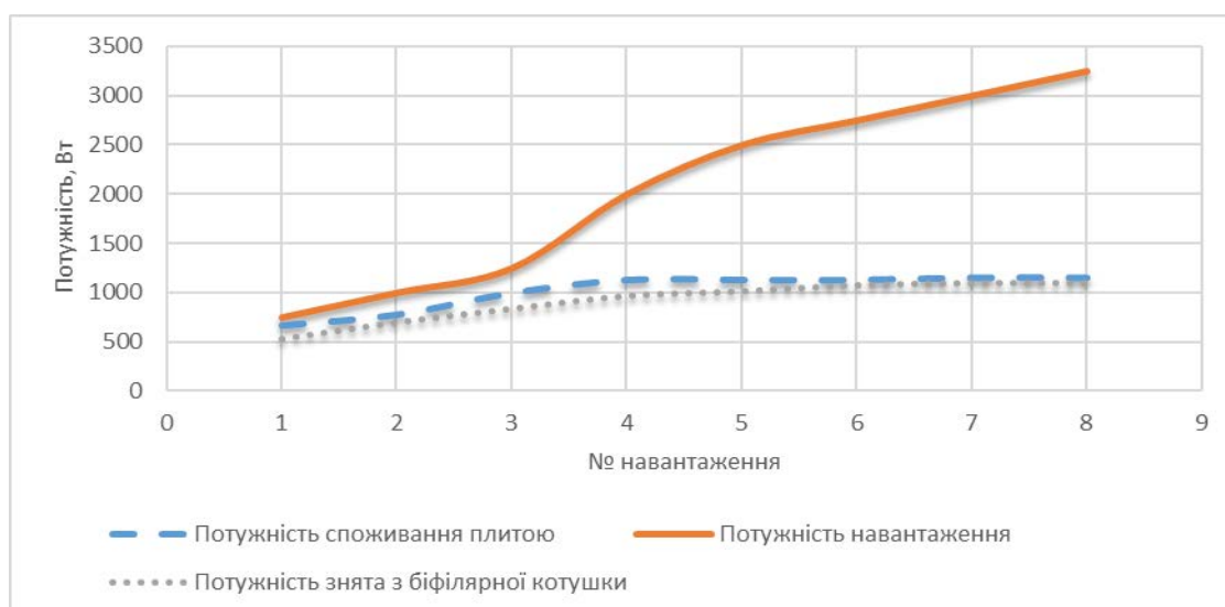
Рис. 1. Графік споживання потужності при використанні двох паралельно з'єднаних біфілярних котушках.
