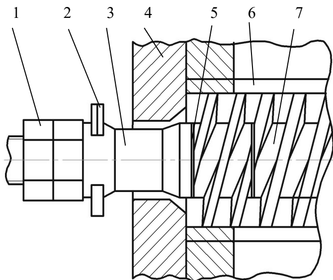
Рис. 1. Фрагмент конструкції конусного зазору в матриці двогвинтових прес- екструдерів: 1 – гайка, 2 – ніж- подрібнювач, 3 – конусна насадка, 4 – матриця, 5 – компенсаційне кільце, 6 – зеерна пластина, 7 – гвинтова насадка.
