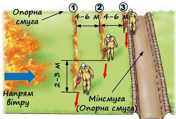
Рис. 9. Контрольований відпал способом випереджувального вогню
