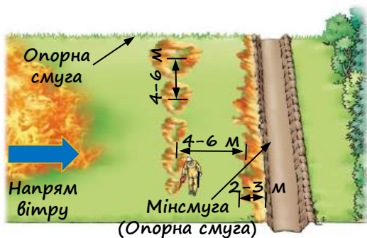
Рис. 10. Відпал способом плямистого відпалу
