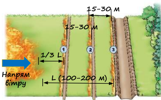
Рис.7. Ступінчастий відпал
