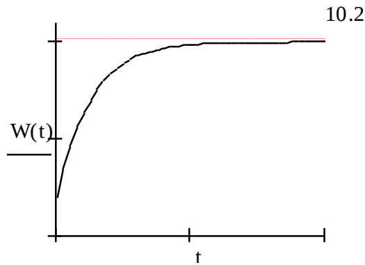
Рис. 3.5. Графік залежності зміни величини маси сухих речовин від часу згідно математичної моделі мономолекулярного росту (мономолекулярне рівняння)
