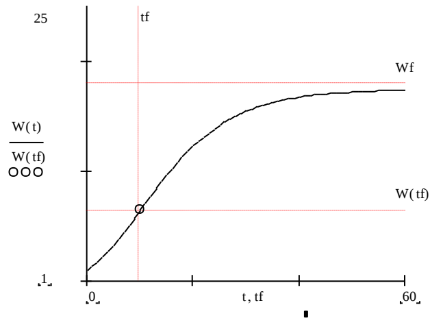
Рис 3.6. Графік залежності зміни величини маси сухих речовин від часу згідно математичної моделі логістичного росту (рівняння логістичного росту)
