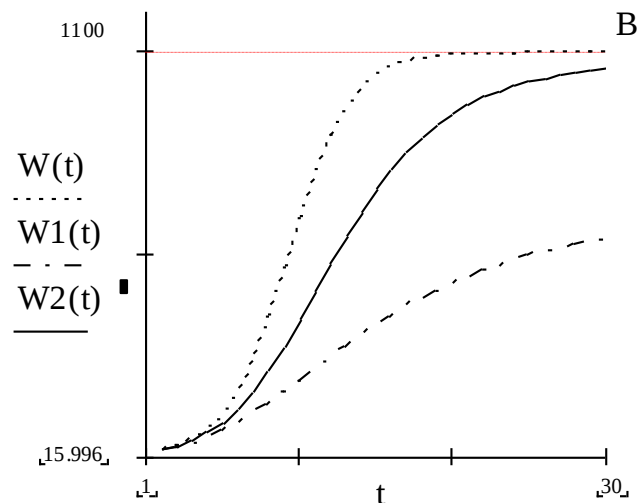
Рис. 3.9. Графік залежності зміни величини маси сухих речовин від часу згідно математичної моделі росту Чантера.
