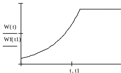
Рис. 3.4. Графік залежності зміни величини маси сухих речовин від часу згідно математичної моделі простого експоненціального росту з різкою відсічкою.
