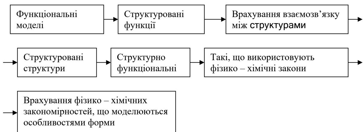
Рис. 3.1. Ієрархія математичних моделей за ступенем відображення властивостей біосистем.
