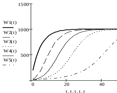
Рис. 3.8. Графік залежності зміни величини маси сухих речовин від часу згідно математичної моделі росту Річардса.
