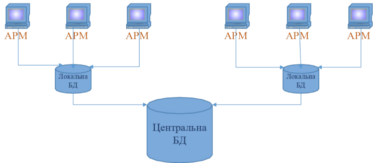
Рис.2 Розподілена система
