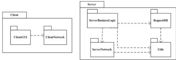
Рис.3 Діаграма пакетів
