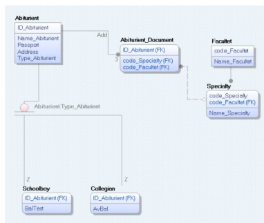
Рис. 1 ER-діаграма
