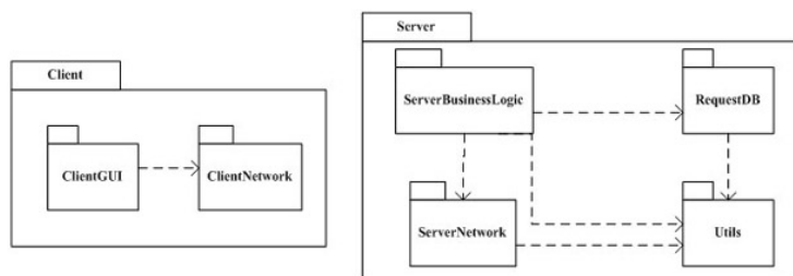
Рис.3 Діаграма пакетів
