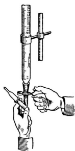
Рис. 2 Видалення повітря з кінчика бюретки;
