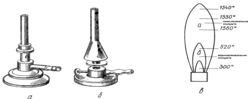
Рис.11. Газові пальники Бунзена (а), Теклю (б) та зони температур полум'я (в)
