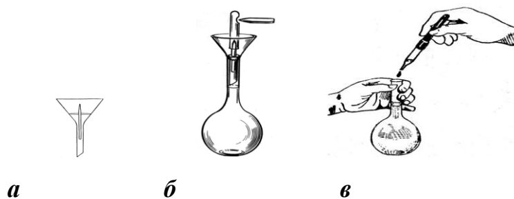
Рис. Приготування титрованого розчину із фіксааналу: а – воронка із скляним бойком; б – розбивання ампул з реактивом; в – остаточне доведення рідини в мірній колбі до мітки.
