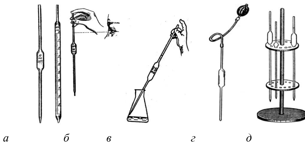
Рис. Мірні піпетки (а): б - положення піпетки для встановлення меніска рідини на рівні риски; в – виливання рідини із піпетки; г – піпетка з гумовою грушею для набирання хімічних реагентів; д – штатив для зберігання піпеток.
