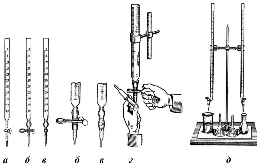
Рис. Бюретки об'ємні для титрування: а – з прямим скляним краном; б – з пружинним металевим затискачем; в – із затискачем у вигляді скляної кульки; г - видалення повітря із кінчика бюретки; д – набір посуду для титрування.
