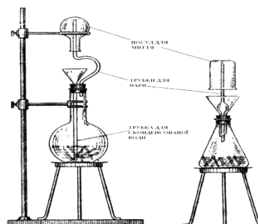
Рис.24. Пристосування для миття та знежирення посуду водяною парою
