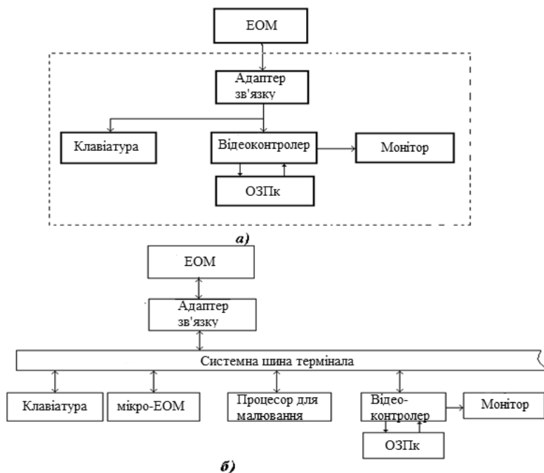
Рис. 1.17. Архітектури графічних систем типу А та В
