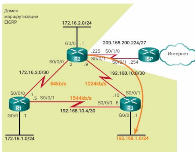
EIGRP для топології IPv4
