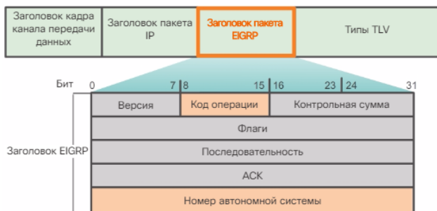
Заголовок пакета EIGRP
