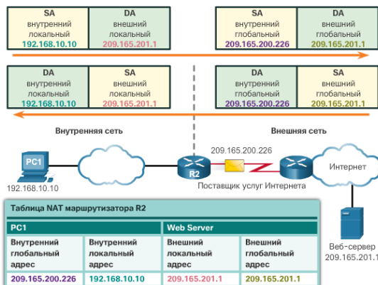
Примеры адресов NAT
