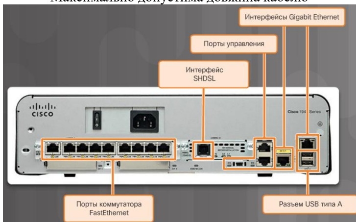
Рис. 1.1.30 Типи інтерфейсів і портів, наявні в маршрутизаторі 1941.
