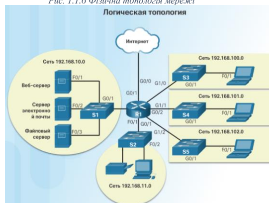
Рис. 1.1.7 Логічна топологія мережі
