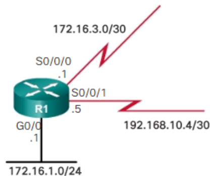
Интерфейсы IPv4 EIGRP
