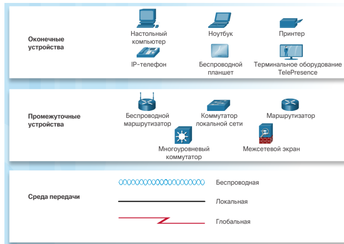
Рис. 1.1.5 Пристрої мережі
