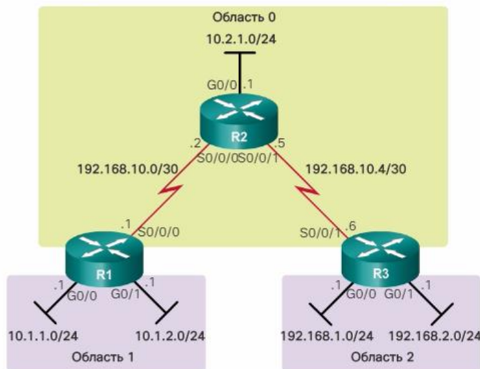
Топологія OSPF для декількох областей
