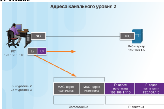
Рис. 1.1.41 Схема адресации каналного уровня
