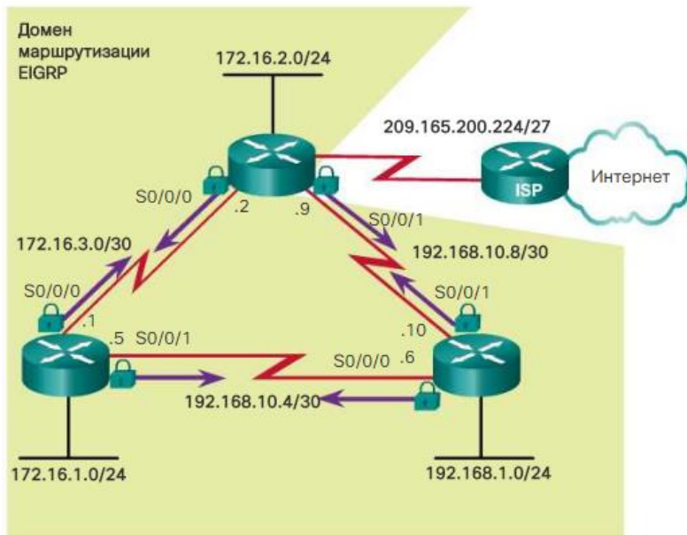
EIGRP для топології IPv4
