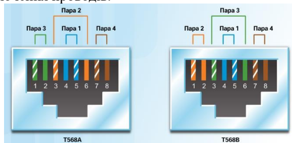
Рис. 1.1.36 Схема обжиму витой пари.
