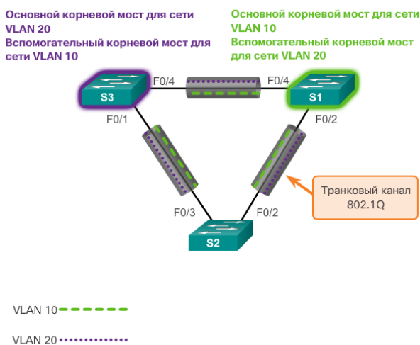
Настройка PVST+
