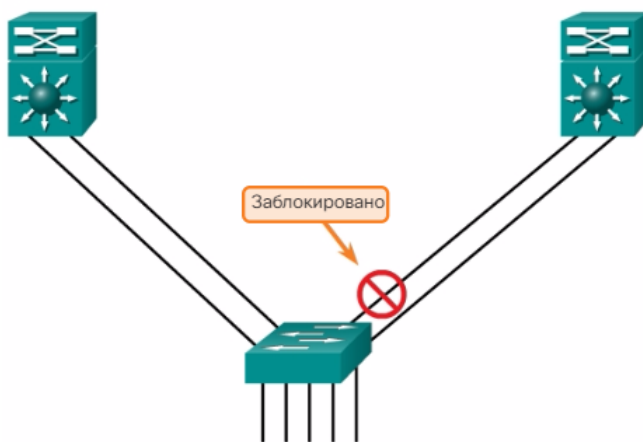
По умолчанию протокол STP блокирует избыточные каналы.
