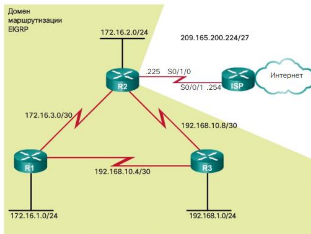
Распространение маршрута по умолчанию
