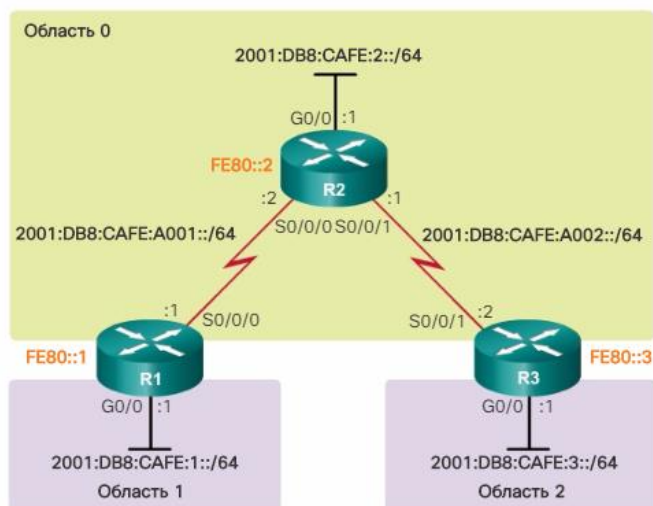
Топологія OSPFv3 для кількох областей
