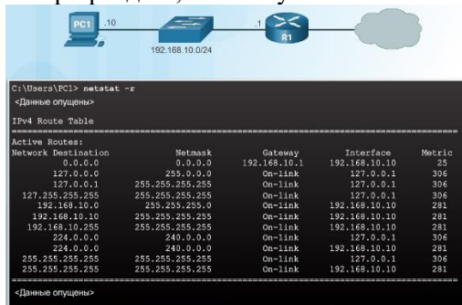
Рис. 1.3.10 Використання утиліти netstat -r
