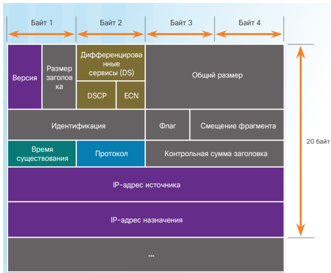
Рис. 1.3.5 Заголовок протокола IPv4
