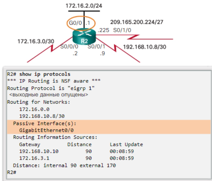
Пассивный интерфейс GigabitEthernet 0/0 маршрутизатора R2
