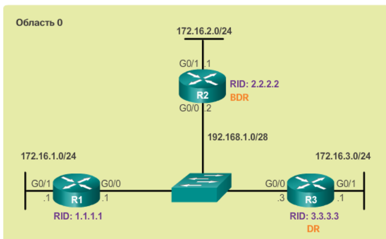
Справочная топология ширококвещательной рассылки OSPF множественного доступа
