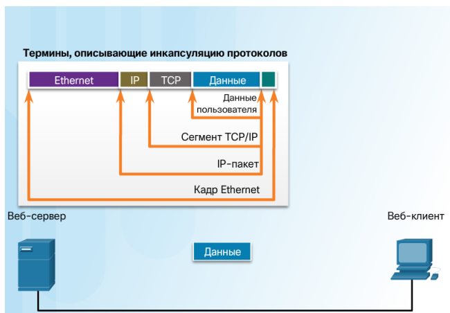
Рис. 1.1.19 Набір протоколів і процес обміну даними
