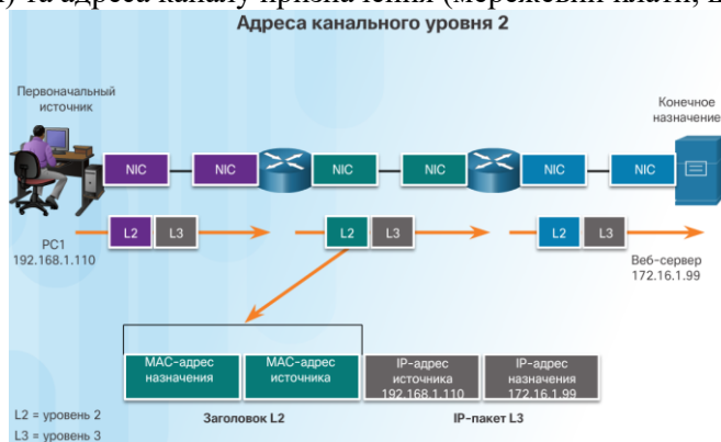
Рис. 1.1.45 Схема адресації на каналному рівні
