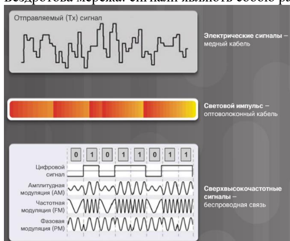
Рис. 1.1.26 Примеры сигналов для медных, оптоволоконных и беспроводных средств подключения
