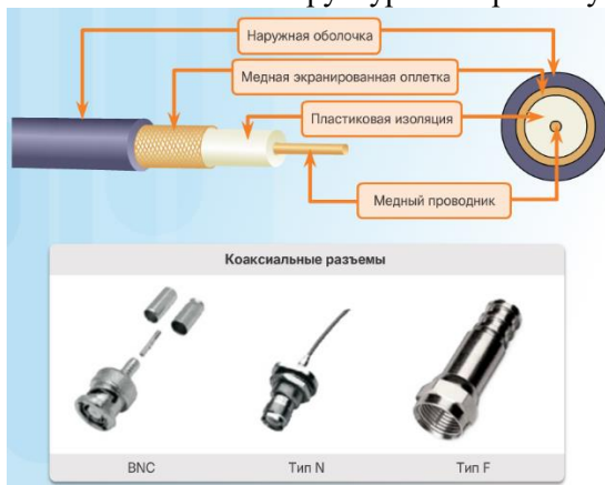
Рис. 1.1.33 Будова коаксіального кабелю
