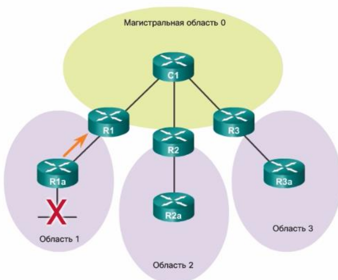
Запрет обновлений с объединением
