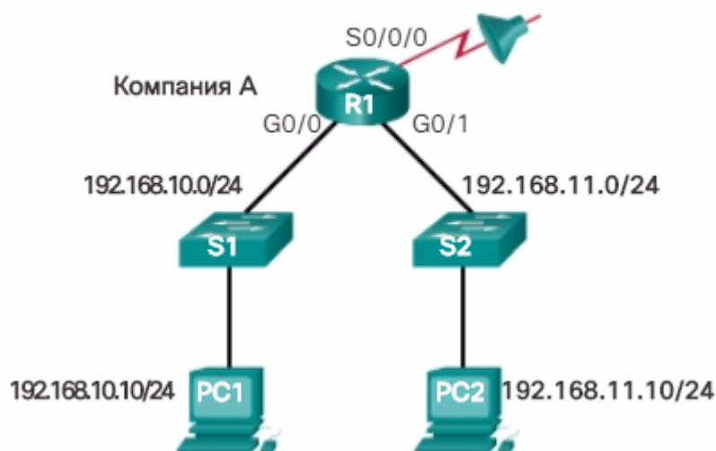
ACL-список 1
