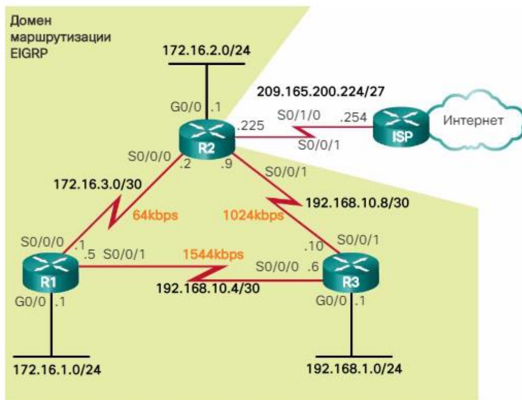
EIGRP для топології IPv4
