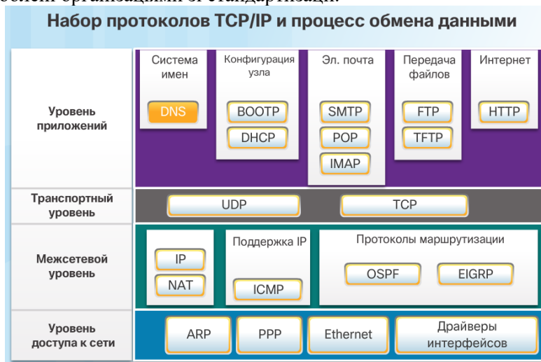
Рис. 1.1.18 Набір протоколів які найбільше застосовуються у мережі
