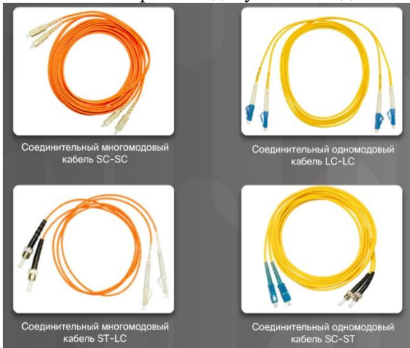
Рис. 1.1.40 Типи з'єднання оптоволоконних кабелів
