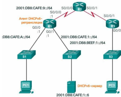
Агент DHCPv6-ретрансляції
