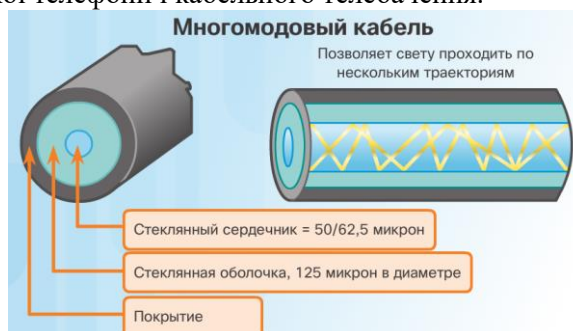
Рис. 1.1.39 Будова багатомодового оптоволоконного кабеля
