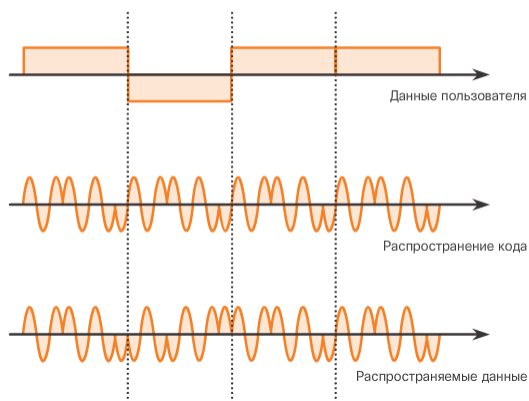
Пример DSSS
