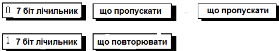
Рис. 3.6. Структури даних при стисненні RLE
