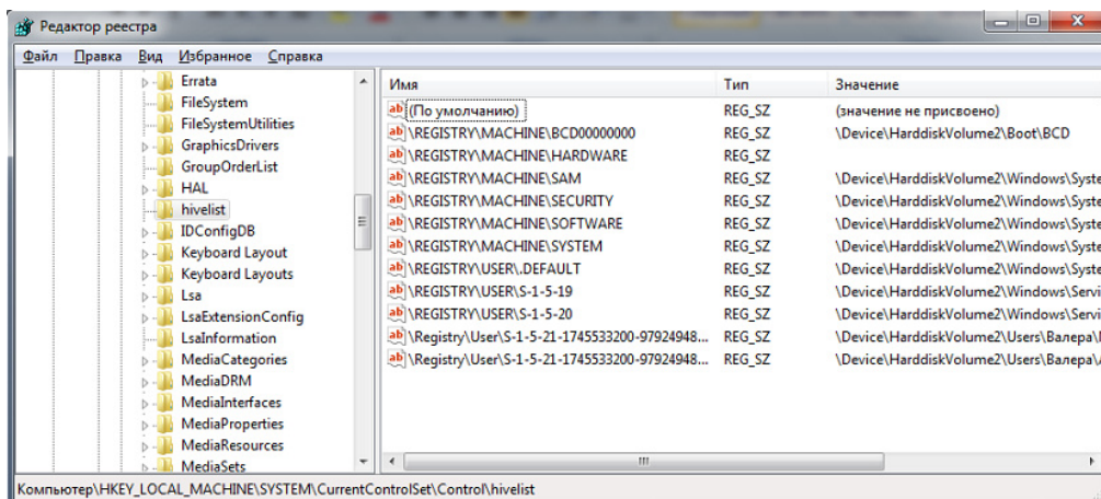
Рис. 2.2. Розділ hivelist з іменами кущів і шляхів до їх каталогів
