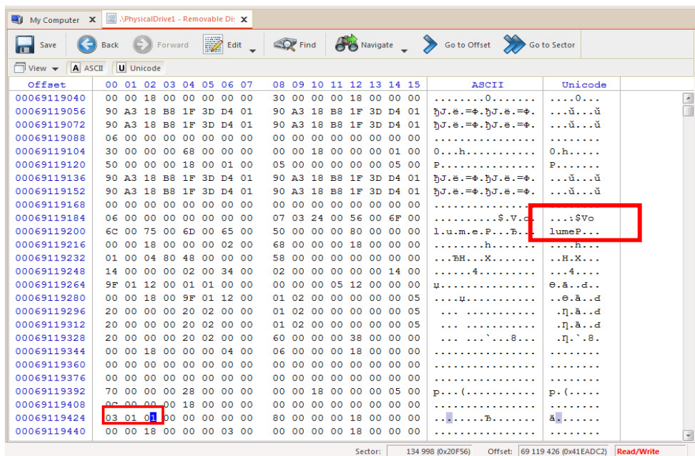
Рис. 1.90. Перехід до службового файлу $Volume
