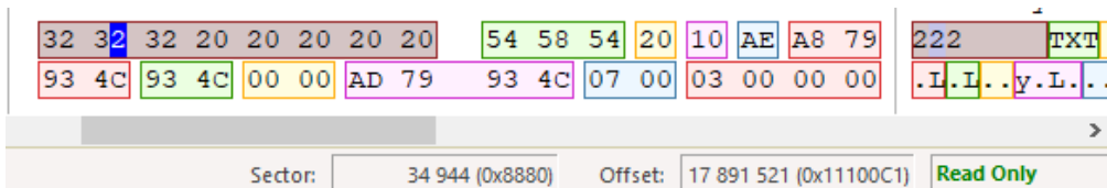
Рис. 1.67. Перехід в сектор запису про файл 2.txt
