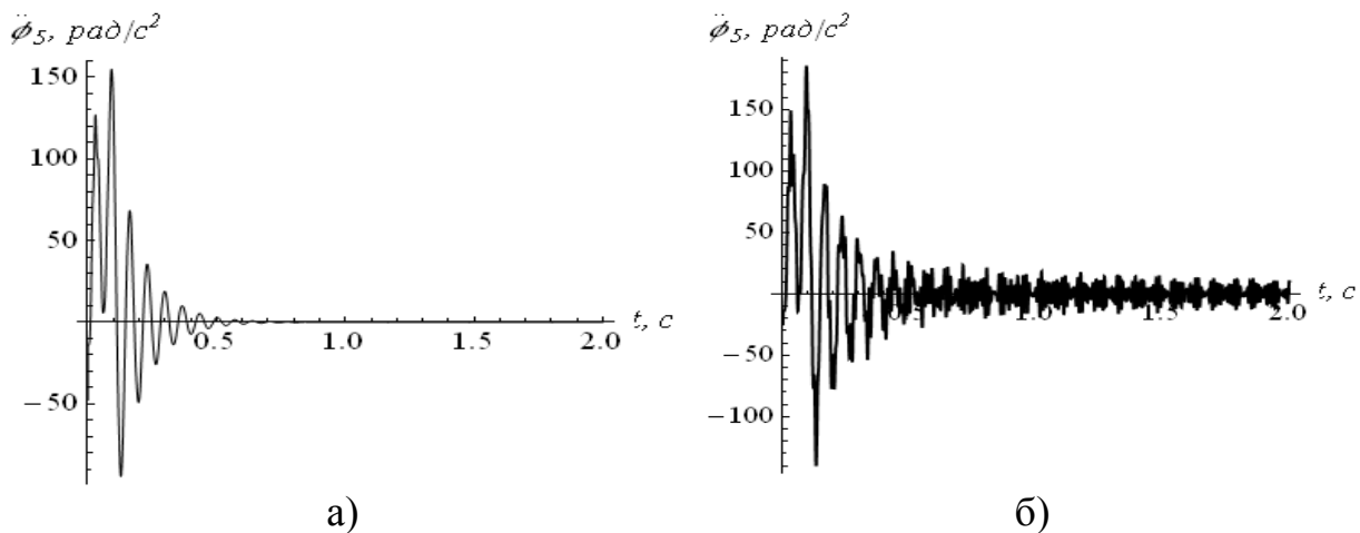
Рис. 5.17. Графіки кутового прискорення \ddot{\varphi}_5 : а) з врахуванням дисипації; б) без врахування дисипації
