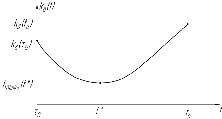
Рис. 3.20. Залежність k_{\partial}(t) (3.240):
