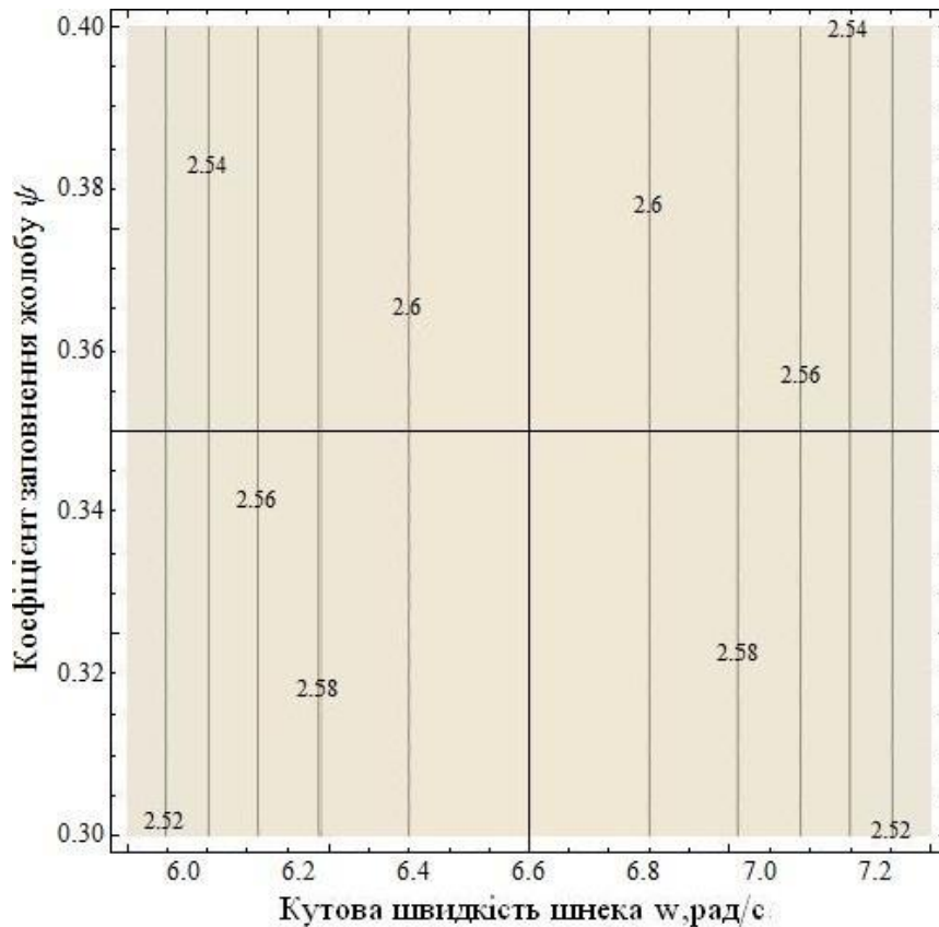
Рис. 7.26 Двомірний перетин поверхні відгуку, що характеризує продуктивність конвєса-змішувача при x_3=0
