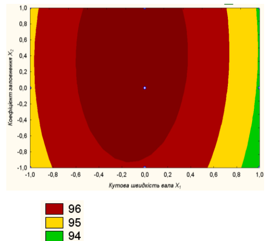
Рис. 7.15. Залежність однорідності від куттової швидкості гвинтового вала і коефіцієнта заповнення жолоба при: а) A = -1 ; б) A = 0 ; в) A = +1
