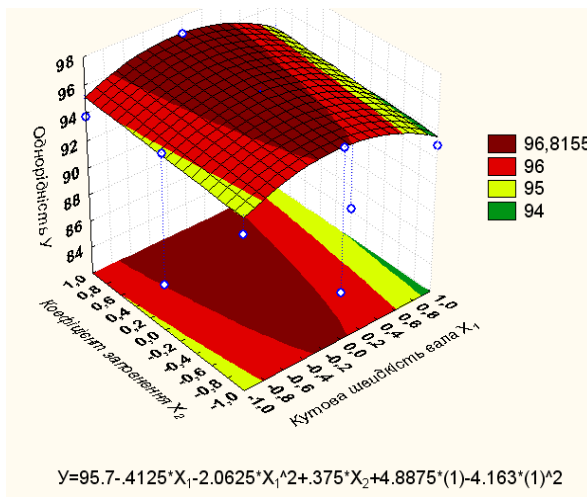
Рис. 7.15. Залежність однорідності від куттової швидкості гвинтового вала і коефіцієнта заповнення жолоба при: а) A = -1 ; б) A = 0 ; в) A = +1
