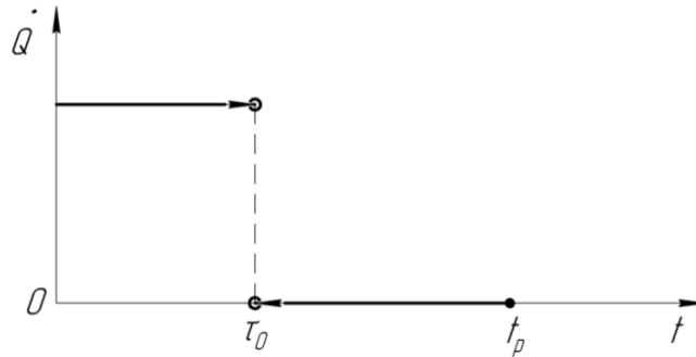
Рис. 3.21. Залежність \dot{Q}(t) .
