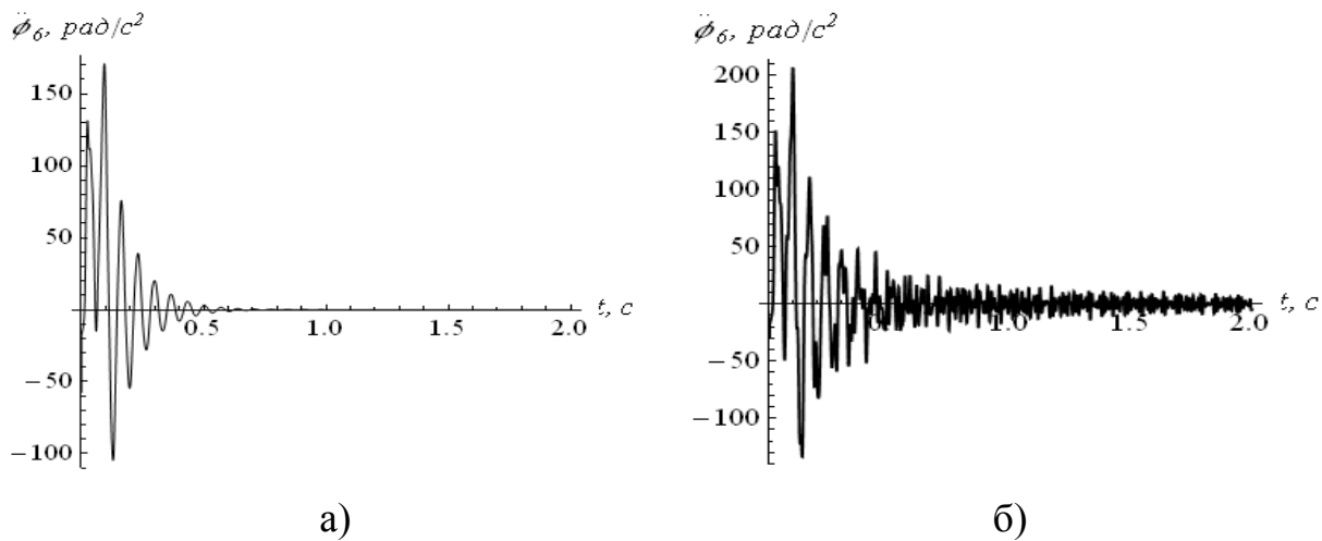
Рис. 5.18. Графіки кутового прискорення \ddot{\varphi}_6 : а) з врахуванням дисипації; б) без врахування дисипації
