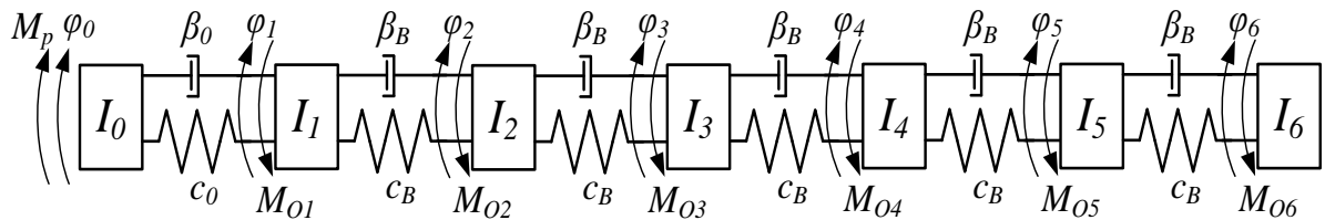
Рис. 4.5. Динамічна модель гвинтового кормозмішувача
