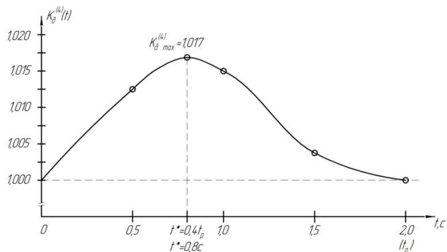
Рис. 3.6. – Залежність K_{\delta}^{(4)}
