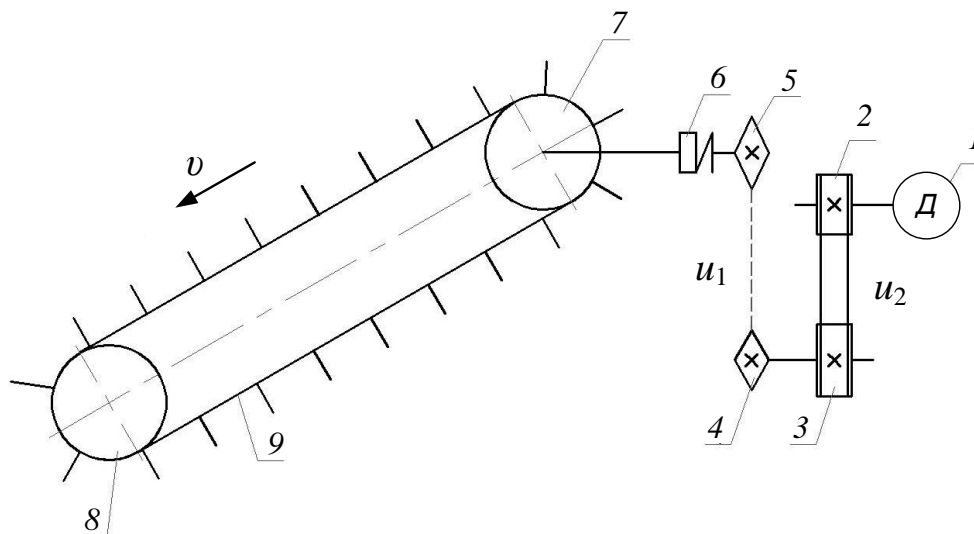
Рис. 4.3. Кінематична схема скребкового конвеєра: 1 – двигун; 2, 3 – шківів пасової передачі; 4, 5 – зірочки ланцюгової передачі; 6 – муфта; 7 – привідна зірочка; 8 – привідна зірочка скребкового конвеєра; 9 – ланцюг зі скребками
