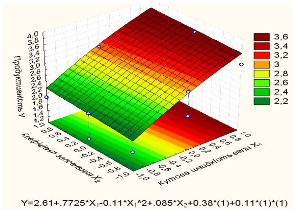
Рис. 7.21. Залежність продуктивності конвеєра-змішувача від кутової швидкості гвинтового вала і коефіцієнта заповнення жолоба при: а) A = -1 ;
