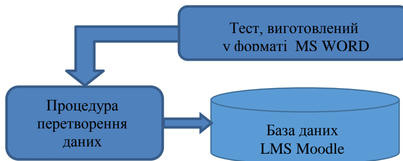
Рис. 1. Структурна схема перетворення тестів із Word у Moodle
